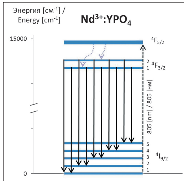
Рис. 1. Диаграмма энергетических уровней иона Nd 3+ в кристалле Nd 3+ :YPO 4 Fig. 1. Diagram of the Nd 3+ energy levels in the Nd 3+ :YPO 4 crystal
