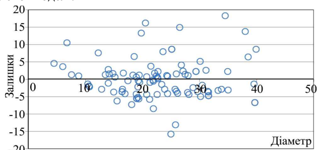
Рис. 2. Дисперсія залишків отриманої функції за діаметром
