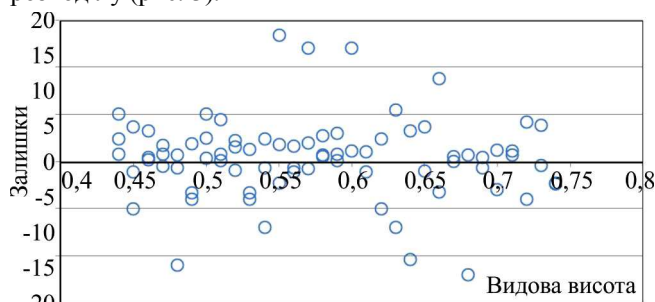
Рис. 3. Дисперсія залишків отриманої функції за числом видової висоти
