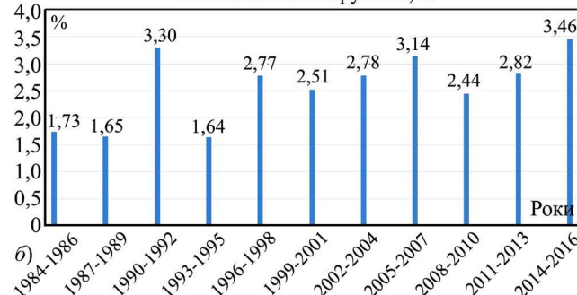
Частка лісових порушень від загальної площі лісу за 3-річчями, % Рис. 3. Загальні показники порушень лісового вкриття в Українських Карпатах: а – річні рівні порушення з 1984 по 2016 рр.; б – частка порушень за кожні три роки
