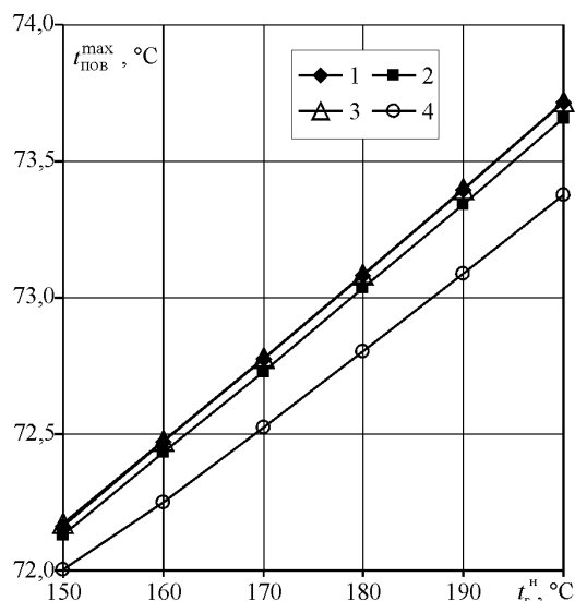
Рис. 3. Залежність максимальної температури t_{\text{пов}}^{\text{max}} поверхні теплообміну водонагрівача від температури t_r^g відхідних газів котла в номінальному режимі котла при застосуванні поверхонь теплообміну із нанокompозитів з різними коефіцієнтами теплопровідності: 1 – \lambda = 30 Вт/(м·К), 2 – 5 Вт/(м·К), 3 – 1 Вт/(м·К), 4 – 0,2 Вт/(м·К)
