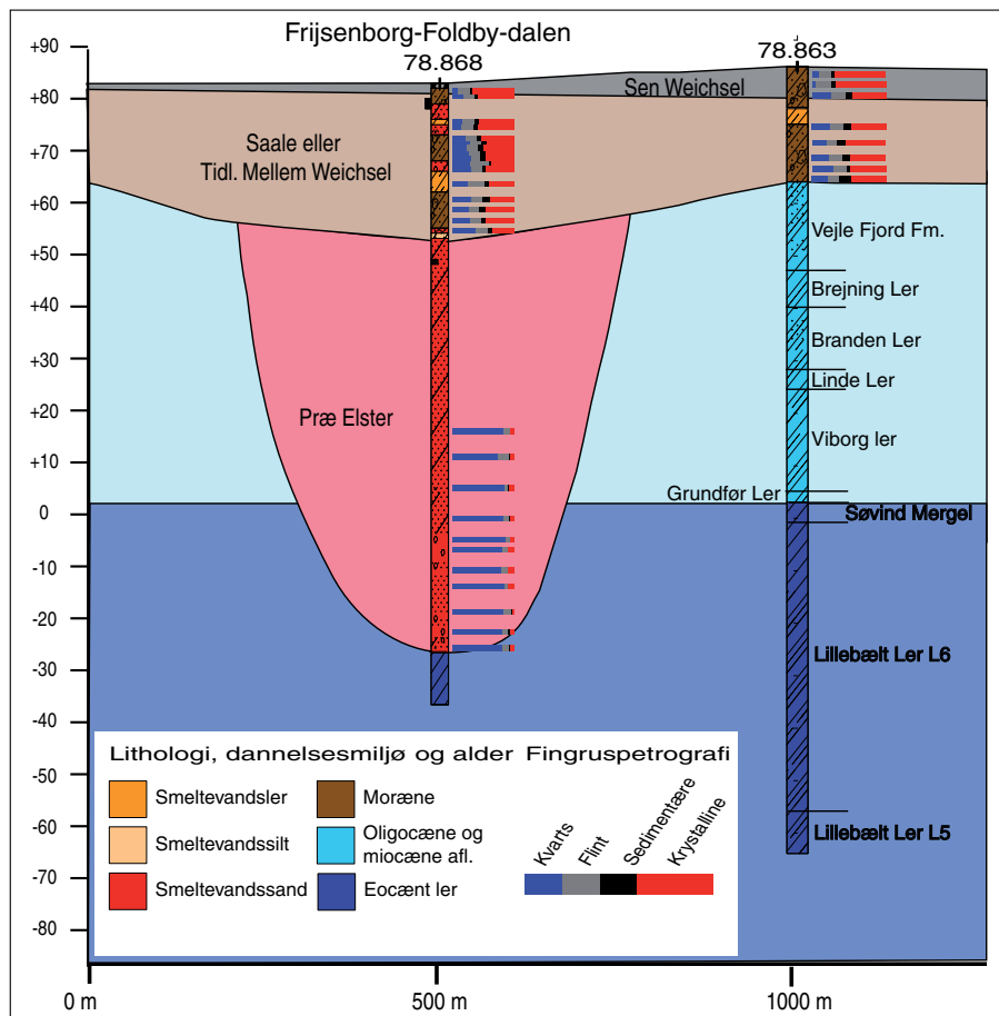
Geologisk snit på tværs af Frijsenborg-Foldby-dalen. (Grafik: Jette Sørensen)
