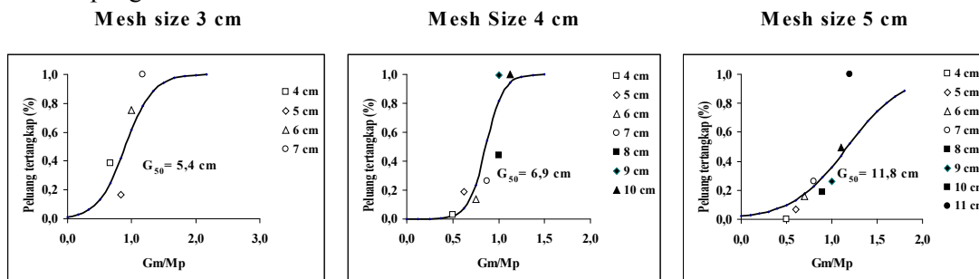
Gambar 3. Kurva selektivitas Sparre-Venema ikan kuniran dari 3 ukuran mata jaring berbeda pada experimental crib alat tangkap sero.
