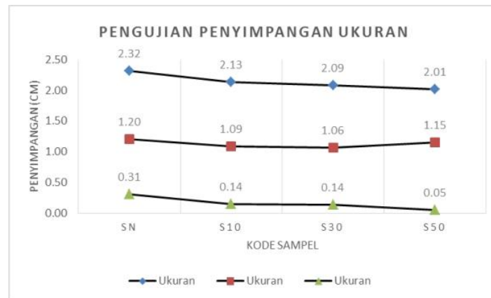
Gambar 7. Grafik Penyimpangan Ukuran
