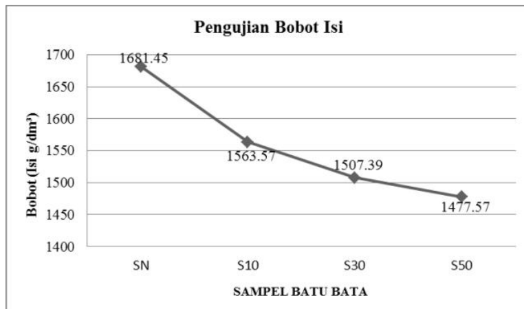
Gambar 8 Grafik Bobot Isi
