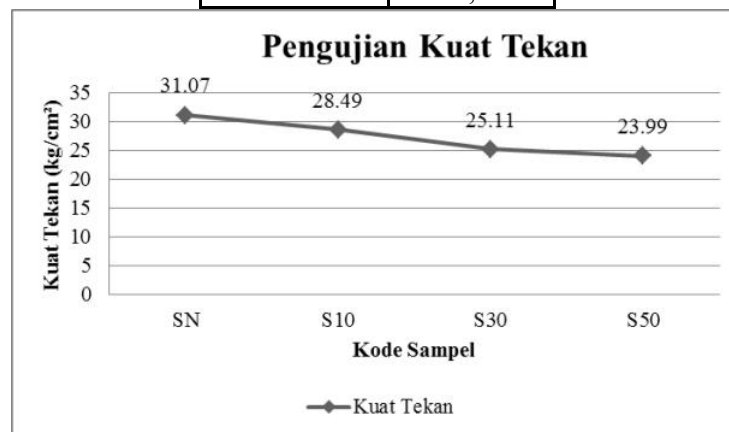
Gambar 11. Grafik Kuat Tekan
