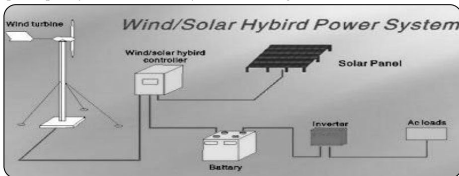
Gambar 1. Hybrid sistem sel surya dan turbin angin
