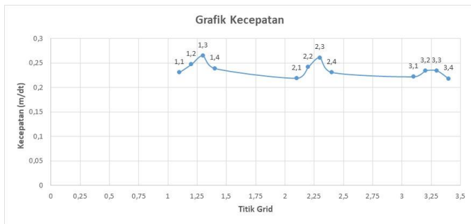
Gambar 9. Grafik kecepatan dasar saluran Kerikil kemiringan 2,5 %
