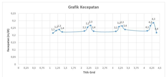
Gambar 9. Grafik kecepatan dasar saluran Kerikil kemiringan 1,5 %
