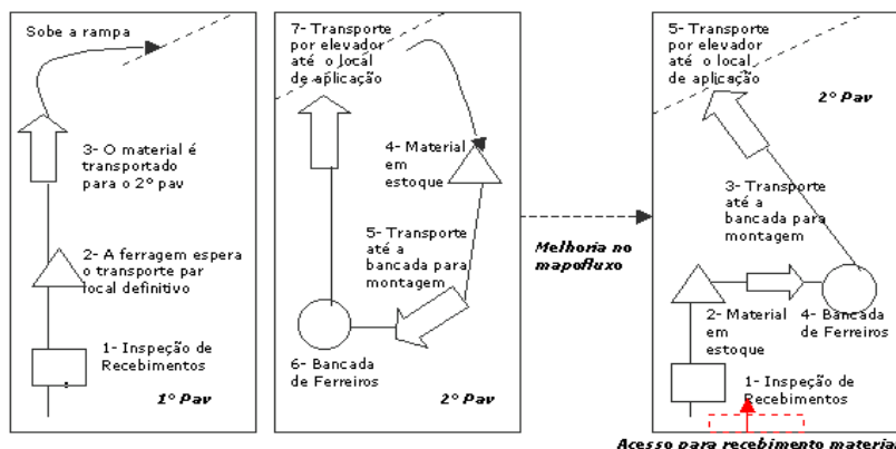
Figura 25 - Mapofluxo do processo de montagem da armadura Fonte: Autores 2012
