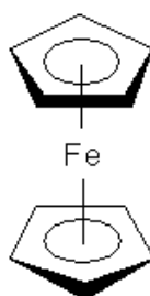
Slika 30. Struktura ferocena
