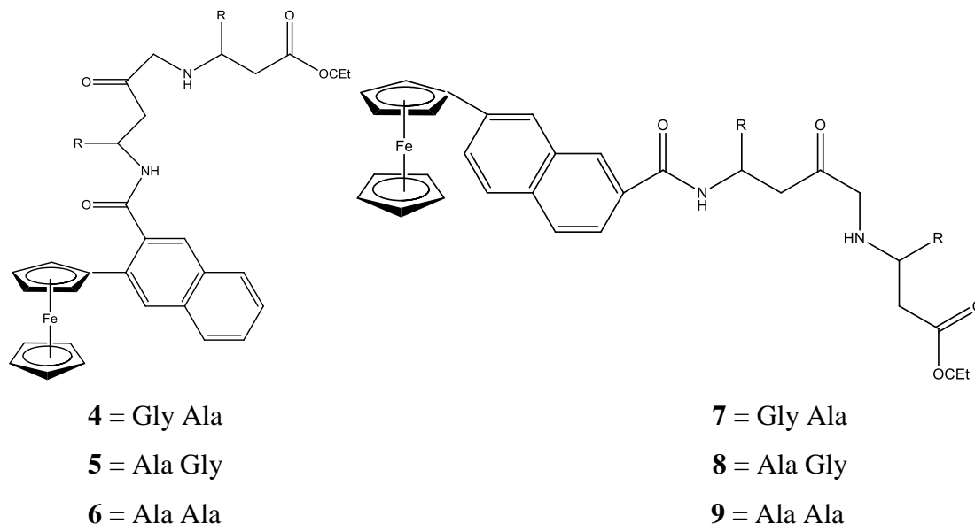
Slika 32. Derivati N-(feroceni)-naftalena
