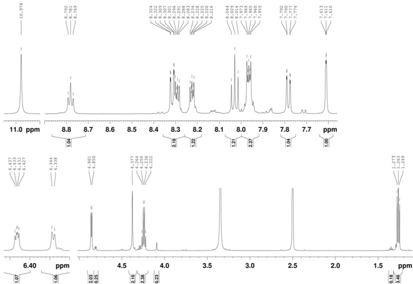
Fig. S23. Expanded ^1\text{H} NMR spectrum of 5e .
