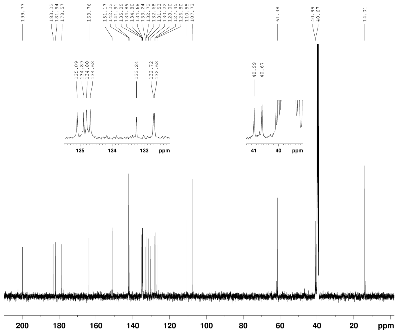
Fig. S24. ^{13}\text{C} NMR spectrum of 5e .
