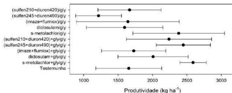
Figura 2. Produtividade de grãos de soja (kg ha -1 ). Embrapa Clima Temperado, 2018/19
