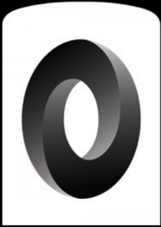
JSON
