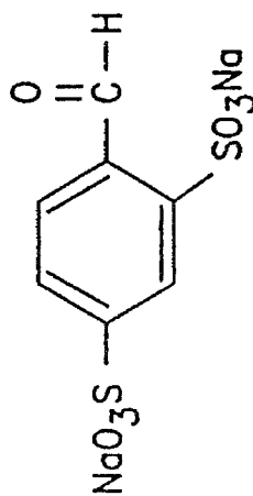
4-Formyl-1,3-benzenesulfonic Acid
