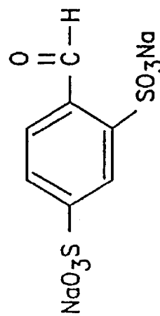
4-Formyl-1,3-benzenesulfonic Acid
