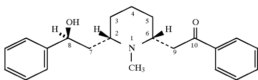
2S,6R,8S(-)Lobeline
