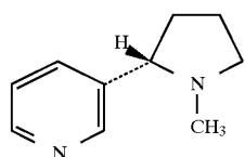
S(-)Nicotine
