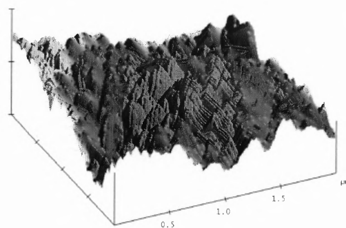
(d) \alpha -Ta 100 \mu\text{m} , R_{\text{rms}} = 22.1 nm
