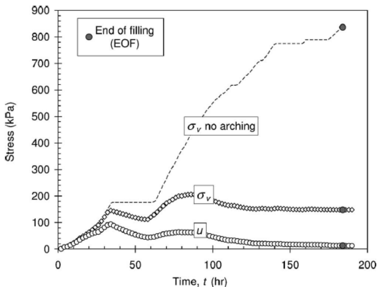
Figure 2–35: Résultats des mesures de pressions à la base du chantier à Kanowna Bell (Helinski et al., 2010)
