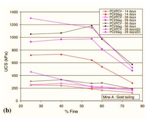
Figure 2–10 Effet du pourcentage des particules très fines sur la résistance du RPC (Fall et Benzaazoua 2005)
