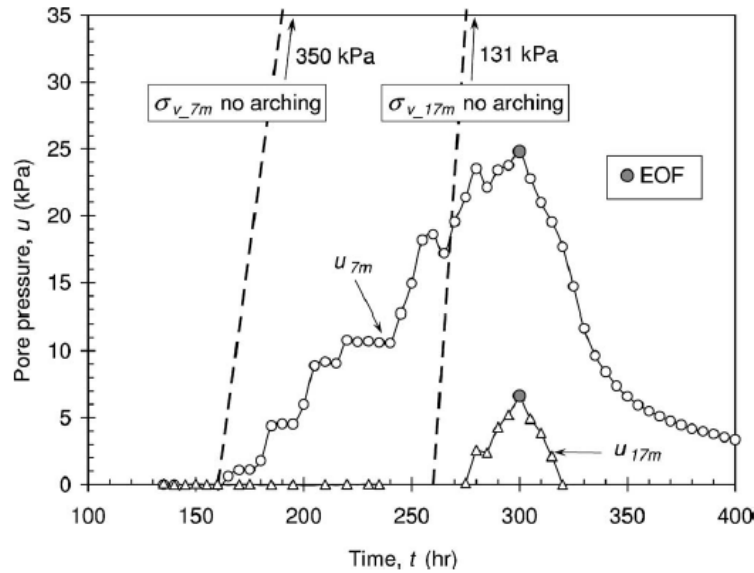
Figure 2–37: Résultats des mesures de pression à la mine Savannah Nickel (Helinski et al., 2010) Après les 300 heures du remblayage, une dissipation de la pression interstitielle du chantier s’est produite. Les pressions maximales enregistrées u_{7m} et u_{17m} tournent respectivement autour de 7 kPa et de 25 kPa. Ce qui est vraiment très faibles comme valeurs.
