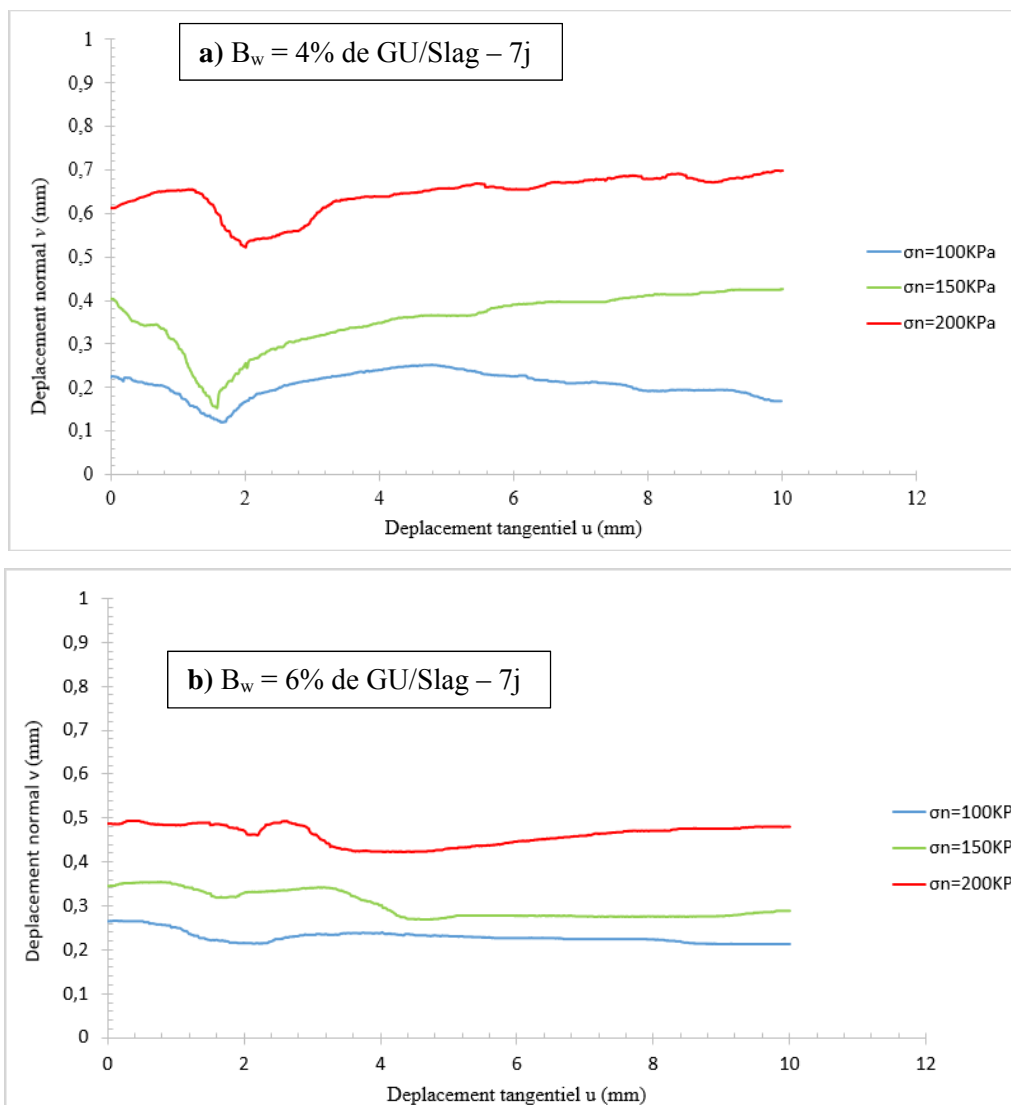
Figure 4–6 Courbes de déplacement normal-déplacement tangential des blocs de remblai curés à 7 jours avec a) 4% de liant, et b) 6% de liant
