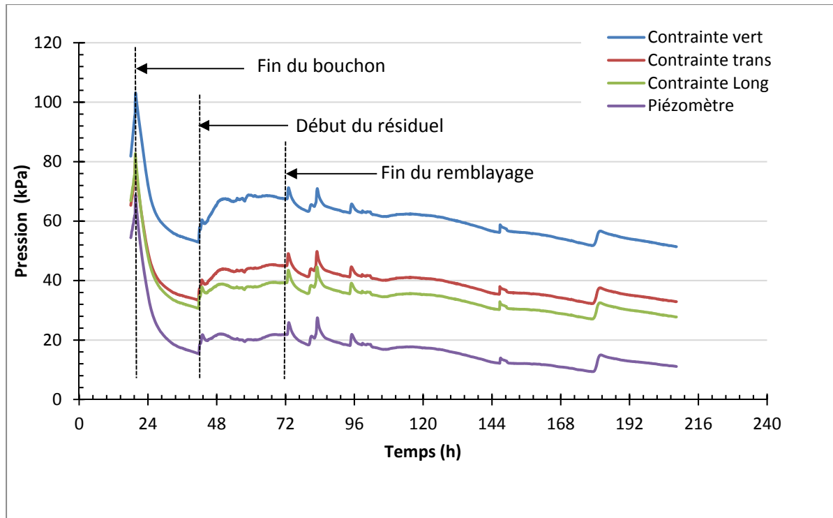
Figure 4–13 : Évolution des pressions dans le chantier #83, 132-03 au 132-04 Z230C (mine Westwood)
