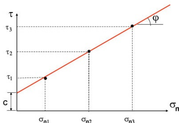
Figure 2–9 Résultat d'un essai de cisaillement direct (droite intrinsèque) dans le plan de Mohr
