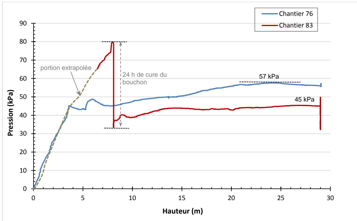
Figure 5-3 : Comparaison des pressions exercées sur la barricade du chantier #76 et du chantier #83
