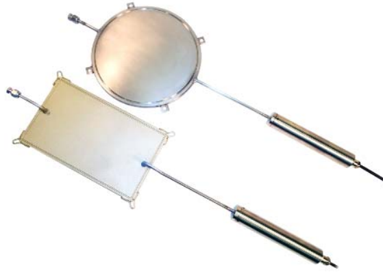
Figure 3–10 Cellules de pression totale (tiré de Roctest)
