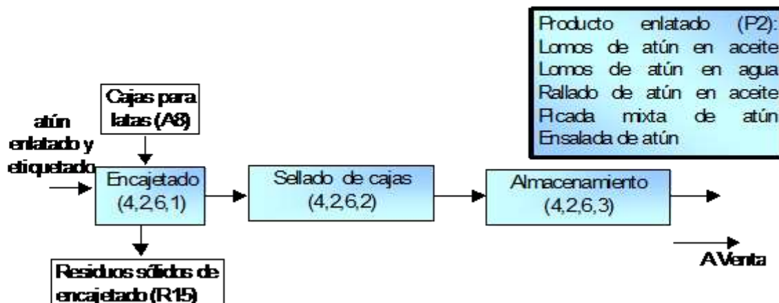
FIGURA 22. Flujograma de Encajetado
