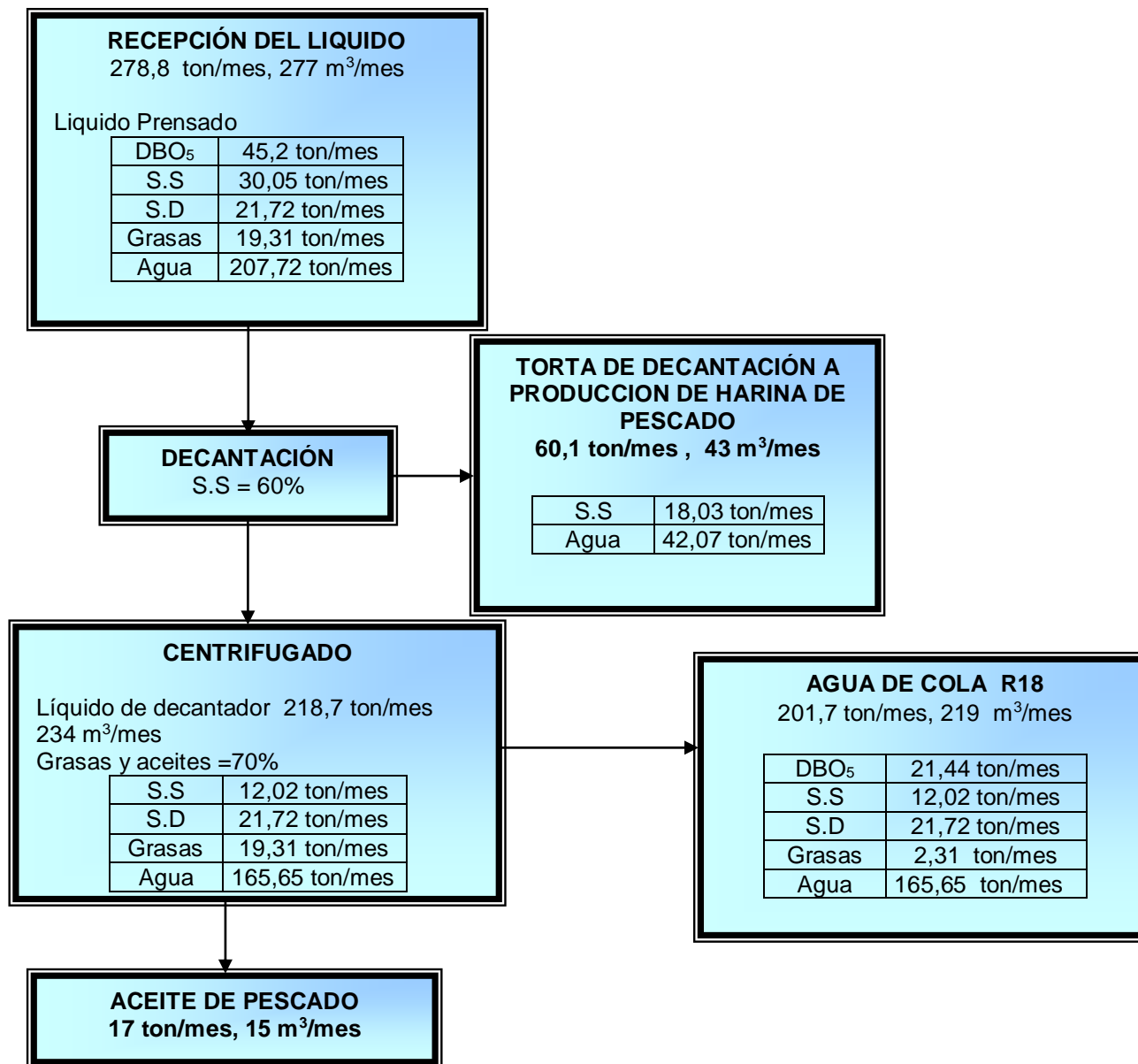
FIGURA 39. Mejoramiento del sistema de decantación en Planta de Subproductos
