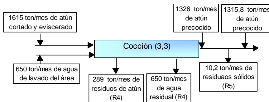
FIGURA 33. Balance de Cocción
