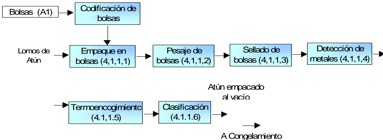
FIGURA 13. Flujograma de Empaque al vacío
