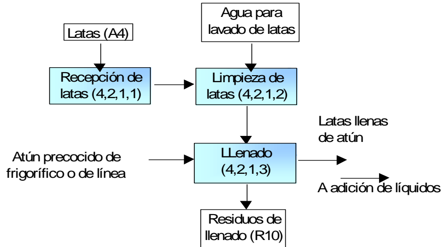
FIGURA 17. Flujograma de Llenado
