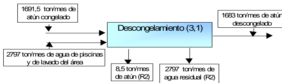
FIGURA 31. Balance de Descongelamiento
