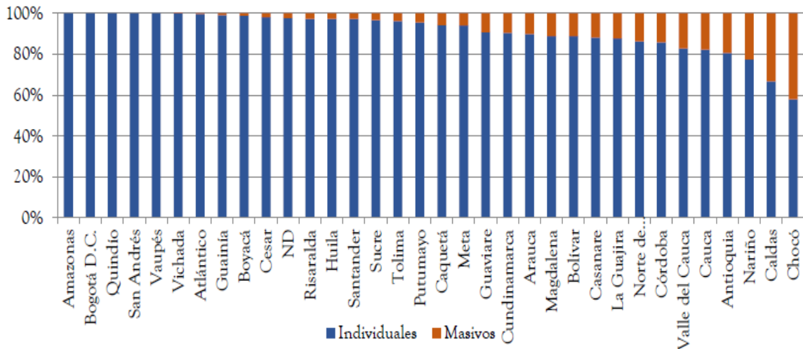
Distribución porcentual de desplazamientos según tipo de desplazamiento
