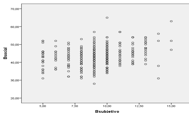
Dispersión entre las variables bienestar Social y bienestar psicológico
