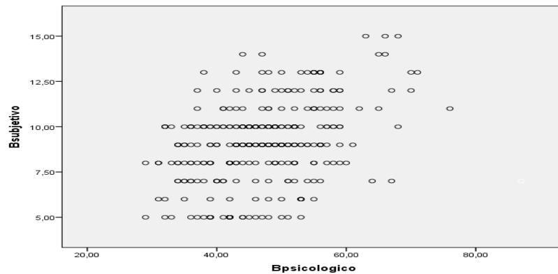
Correlación Variables Bsubjetivo y Bpsicologico. SPSS versión 18.0
