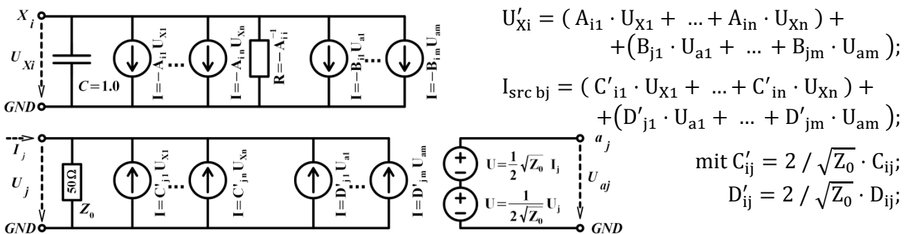
Abb. 3: Schaltkreis in einer Streuungsform („S-Parameter“) a) Schaltkreis für i ten internen Zustand b) Schaltkreis für j ten Port (Einspeisen der gestreuten Welle und Berechnen der einkommenden Welle)
