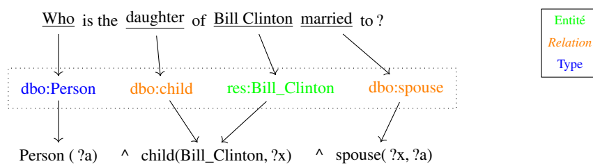
Figure 2. Analyse de la question et construction de la requête
