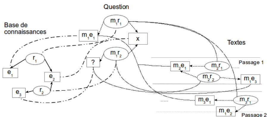
Figure 3. Recherche de réponses dans une base de connaissances ou dans les textes
