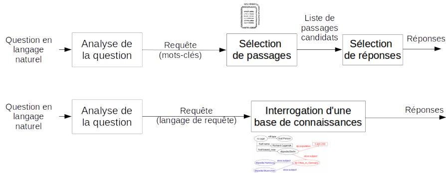
Figure 1. Architecture de recherche de réponses à partir de questions en langage naturel
