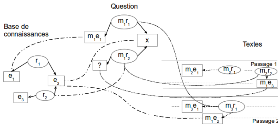
Figure 4. Hybridation du processus de recherche
