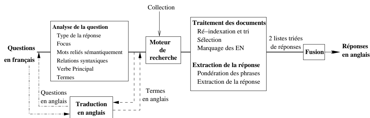
FIG. 1 – Architecture du système de question-réponse multilingue
