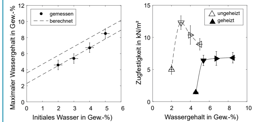
Bild 4: a) Maximaler auftretender Wassergehalt im Prüfkörper bei der Nasszugfestigkeitsprüfung, aufgetragen gegen den initialen Wassergehalt im noch ungeheizten Formsand. Der berechnete Zusammenhang basiert auf einer Wärmekapazität von 0,84 bzw. 1,26 kJ/kg K für die untere bzw. obere Gerade. b) Zugfestigkeiten der ungeheizten feuchten Formsande (offene Dreiecke) und die dazugehörigen (geheizten) Nasszugfestigkeiten, aufgetragen über dem Wassergehalt an der Bruchstelle (Dreiecke mit gleicher Orientierung gehören zu den gleichen Sanden). (Abbildung modifiziert aus [27])
