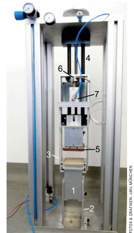
Bild 1: Neutronenstrahlkompatible Nasszugfestigkeitsprüfapparatur für Formsande: (1) quadratischer Prüfkörperbehälter, (2) Prüfkörperaufnahme, (3) Zuggestänge mit Haken zum Aufbau einer Zugspannung am Prüfkörperkopf, (4) mechanisch betriebene Spindel zur Grobpositionierung des Zuggestänges, (5) Stirrheizung, (6) Drucksensors, (7) pneumatischer Druckzylinder.
