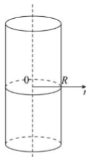
Рисунок 2.3 – Геометрия области решения
