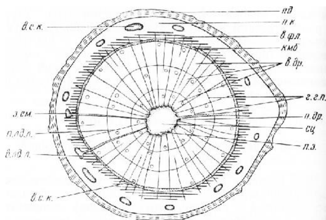
Рисунок 2.1. – строение еловой ветви
