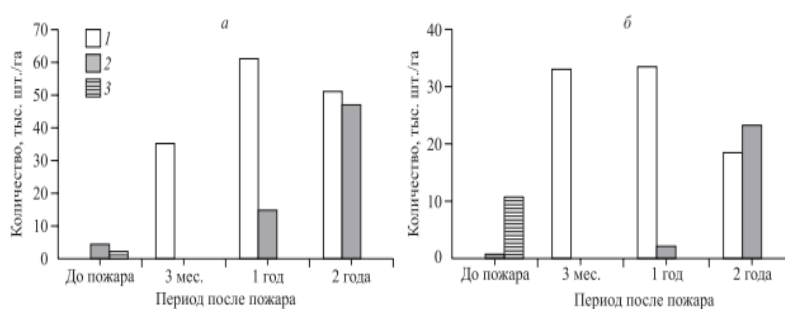
Рис. 4 [52]. Динамика возобновления в сосновых насаждениях до и после экспериментальных выжиганий; а – средневозрастное насаждение; б – спелое насаждение; 1 – всходы; 2 – самосев; 3 – подрост
