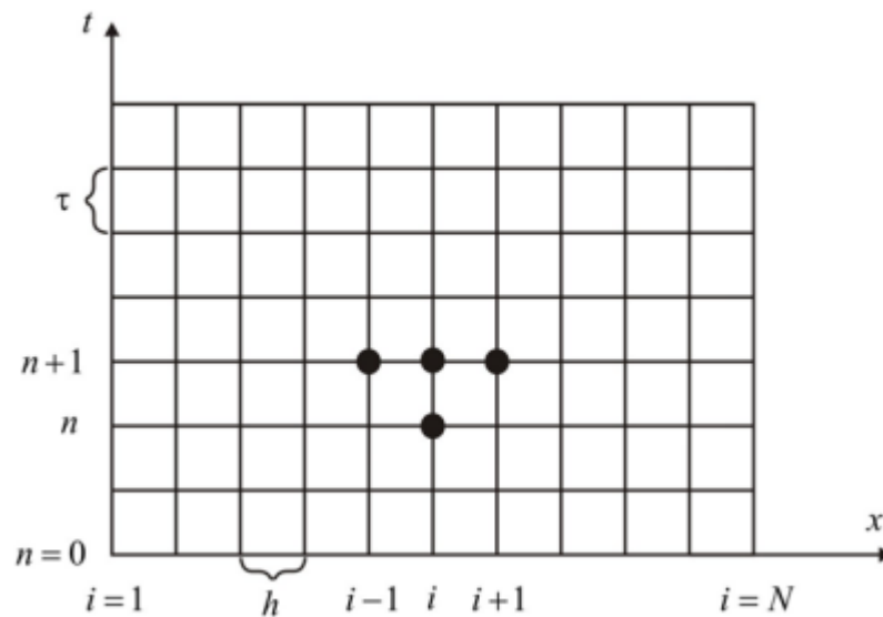
Рисунок 2.1-Шаблон неявной разностной схемы [1]
