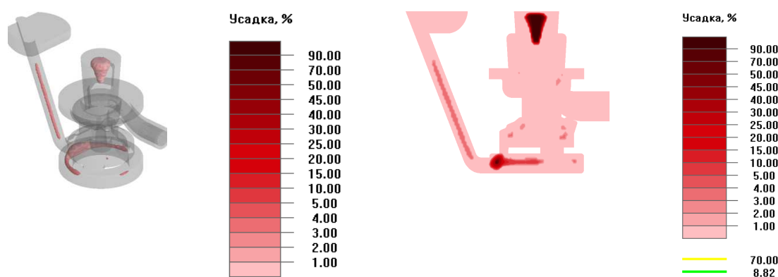
Рис. 5. Анализ усадки
