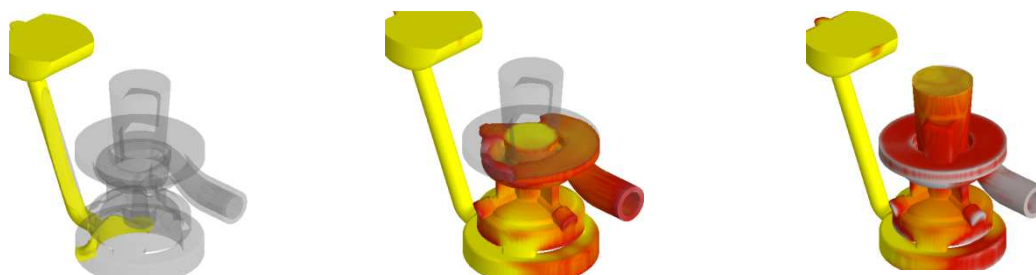
Рис. 3. Процесс заполнения кокиля сплавом
