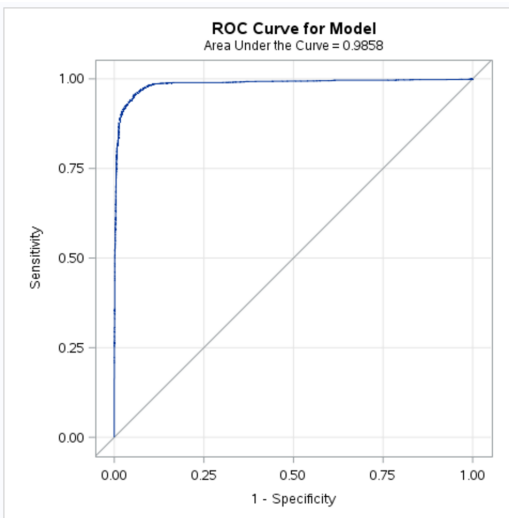
Fig. 12: ROC Index and AUC Index for LA
