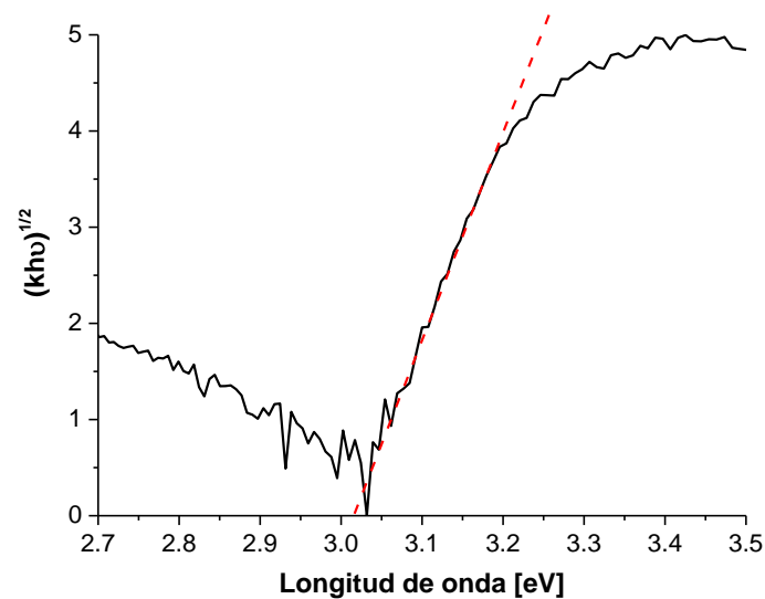
Figura 3.24: Gráfica Tauc de la probeta S4-V120-J500-t5-TT.
