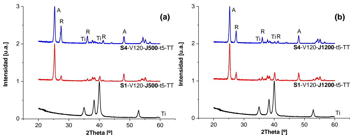
Figura 3.36: Difractogramas normalizados. Influencia de la concentración del electrolito. Sustrato (Ti) y probetas (a) S1-V120-J500-t5-TT y S4-V120-J500-t5-TT y (b) S1-V120-J1200-t5-TT y S4-V120-J1200-t5-TT . A: anatasa; R: rutilo; Ti: titanio.
