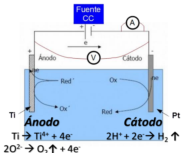
Figura 3.17: Esquema de la celda electroquímica utilizada en las anodizaciones y reacciones en ánodo y cátodo.
