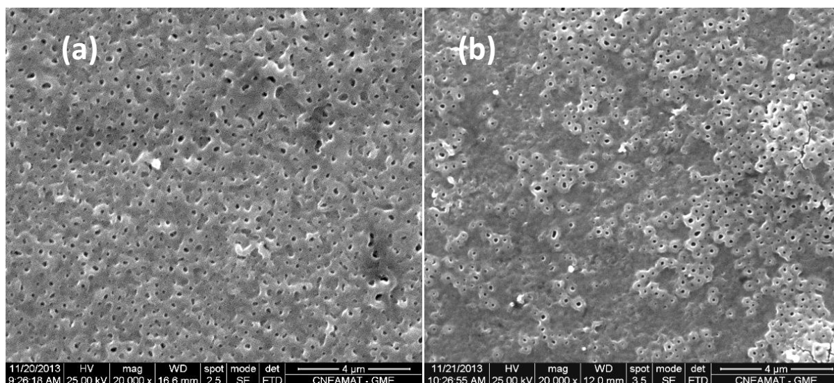
Figura II.3: Micrografías electrónicas. Influencia de la temperatura del electrolito. Probetas (a) S0,5-V150-J500-t5- T25 y (b) S0,5-V150-J500-t5- T40 .
