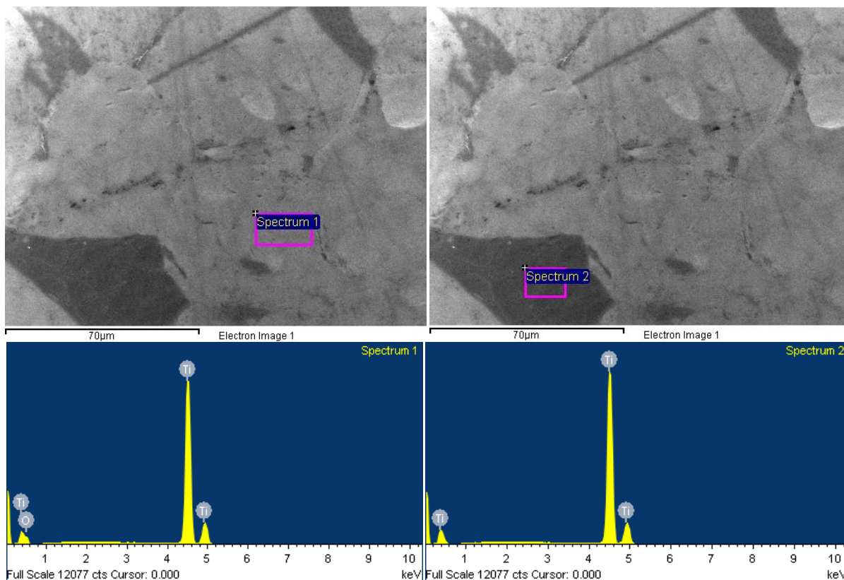
Figura 4.8: Micrografías electrónicas con EDS. Influencia de la textura del sustrato. Probeta Probeta HF-V20-t120-TT. Izquierda: zona clara. Derecha: zona oscura.
