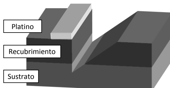
Figura 3.11: Diagrama de la muesca realizada por FIB-MEB.
