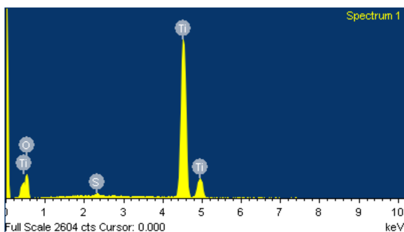
Figura 3.22: Análisis composicional de la probeta S4-V120-J1200-t5-TT.
