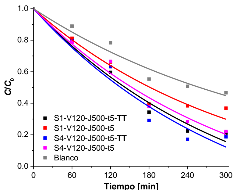
Figura III.4: Perfiles temporales de concentración normalizada de Cr(VI) ( C/C_0 ) para la reacción fotocatalítica en presencia de EDTA con las probetas S1-V120-J500-t5-TT, S1-V120-J500-t5, S4-V120-J500-t5-TT y S4-V120-J500-t5. Condiciones experimentales: [K_2Cr_2O_7] = 0,4 \text{ mM} , [EDTA] = 1 \text{ mM} , \text{pH } 2 , E_{365\text{nm}} = 3700 \text{ } \mu\text{W}/\text{cm}^2 , T = 25 \text{ } ^\circ\text{C} . Las líneas representan el ajuste de las curvas con la ecuación 3.4
