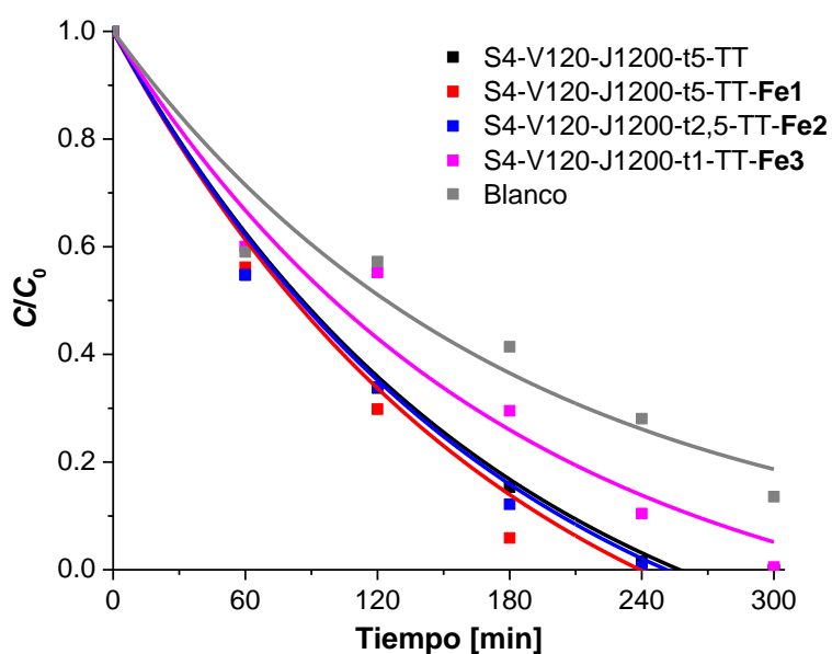
Figura 3.60: Perfiles temporales de concentración normalizada de Cr(VI) ( C/C_0 ) para la reacción fotocatalítica en presencia de EDTA con las Probetas de referencia y probetas S4-V120-J1200-t5-Fe1, S4-V120-J1200-t2,5-Fe2 y S4-V120-J1200-t1-Fe3. Condiciones experimentales: [\text{K}_2\text{Cr}_2\text{O}_7] = 0,4 \text{ mM} , [\text{EDTA}] = 1 \text{ mM} , \text{pH } 2 , E_{365\text{nm}} = 5750 \mu\text{W}/\text{cm}^2 , T = 25 \text{ }^\circ\text{C} . Las líneas representan el ajuste de las curvas con la ecuación 3.4.
