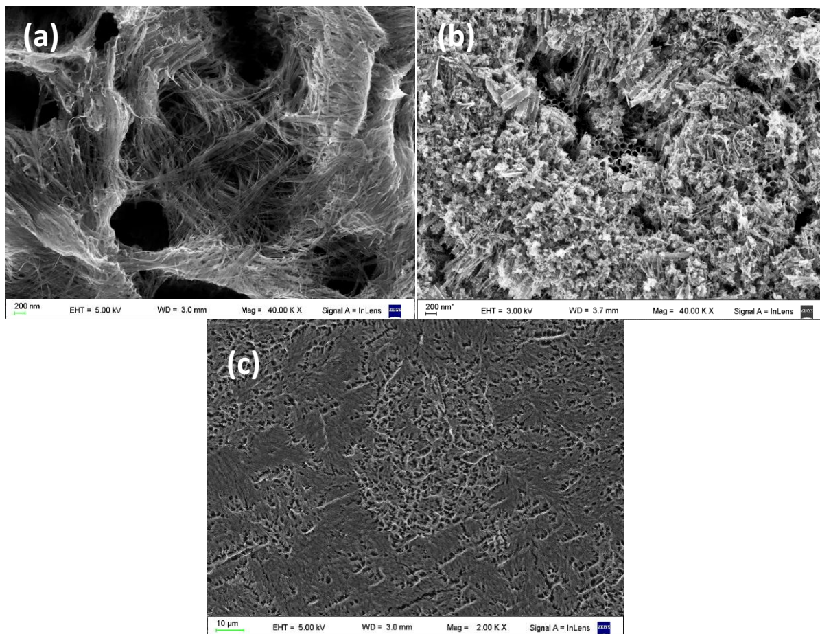
Figura 5.3: Micrografías electrónicas. Nanopastos obtenidos durante la síntesis de NTL. (a) EG-V60-t2, (b) EG-V45-t2-TT y (c) EG-V60-t2-TT-450-2.
