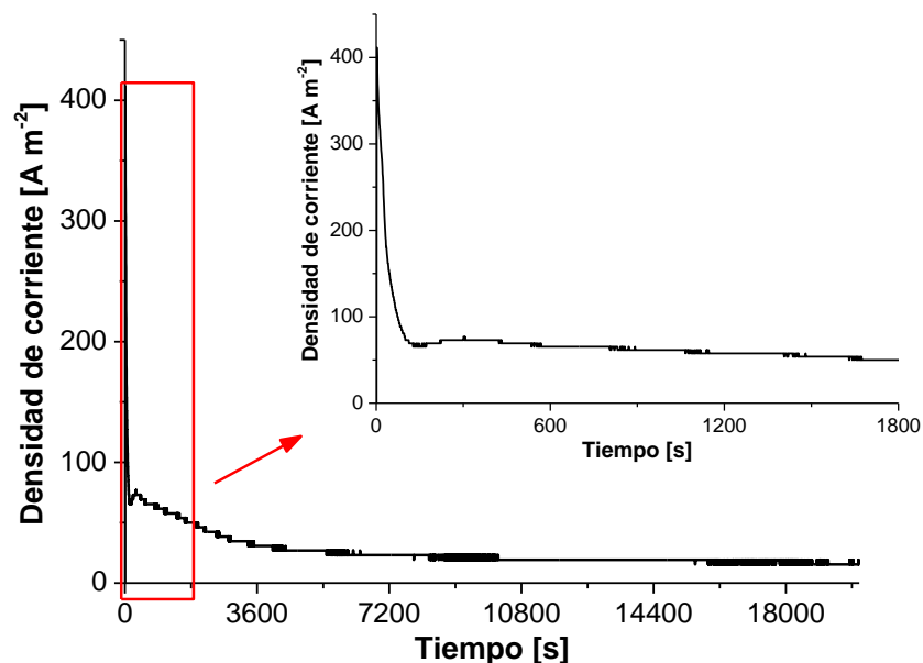
Figura 5.14: Evolución temporal de la densidad de corriente. Probeta EG-V45- t8 -TT-450-2.
