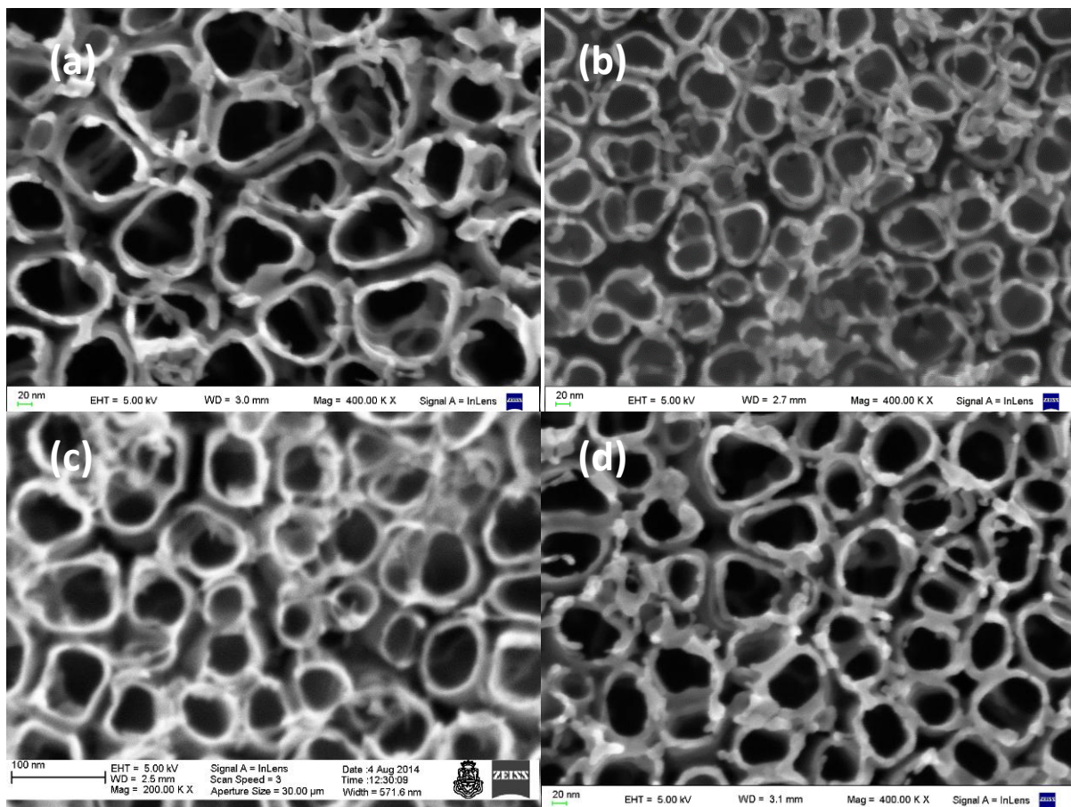
Figura 4.17: Micrografías electrónicas. Influencia del tiempo de anodización. Probetas (a) HF-V20-t5-TT, (b) HF-V20-t15-TT, (c) HF-V20-t30-TT y (d) HF-V20-t120-TT.
