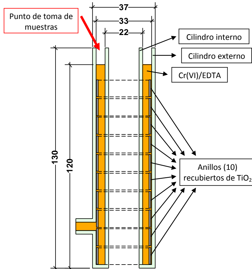
Figura 6.8: Representación de reactor, con anillos recubiertos y solución de Cr(VI)/EDTA. Corte longitudinal. Dimensiones en mm. La flecha roja indica el punto de toma de muestra.
