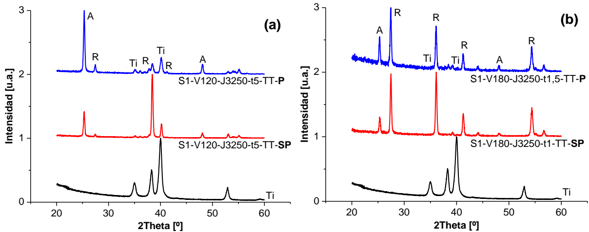
Figura I.5: Difractogramas normalizados. Influencia de la preparación superficial. Sustrato (Ti) y probetas (a) S1-V120-J3250-t5-TT-P y S1-V120-J3250-t5-TT-SP y (b) S1-V180-J3250-t1,5-TT-P, S1-V180-J3250-t1-TT-SP. A: anatasa; R: rutilo; Ti: titanio.
