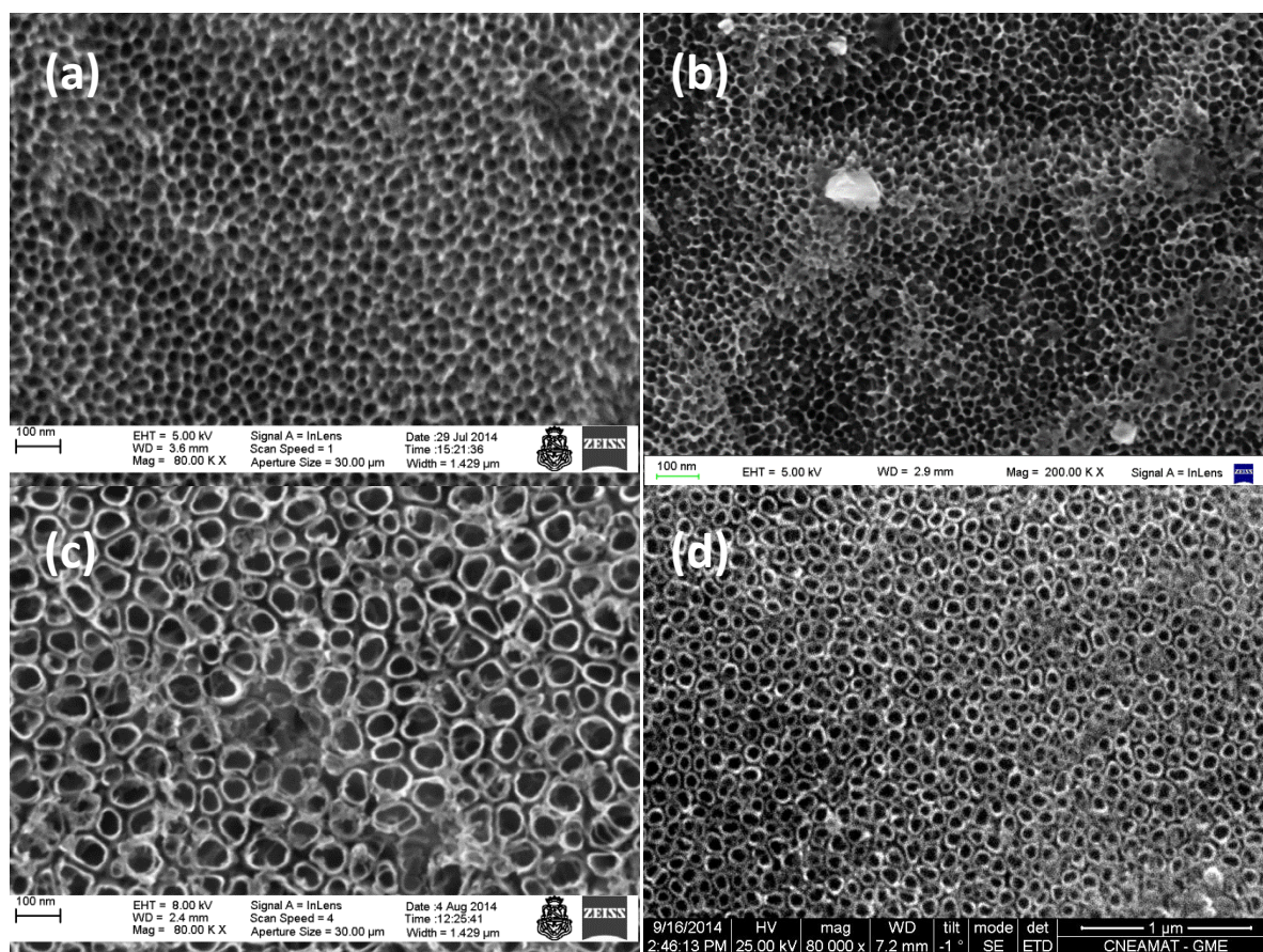
Figura 4.13: Micrografías electrónicas. Influencia del voltaje. Probetas (a) HF- V8 -t15-TT, (b) HF- V12 -t15-TT, (c) HF- V15 -t15-TT y (d) HF- V20 -t15-TT.
