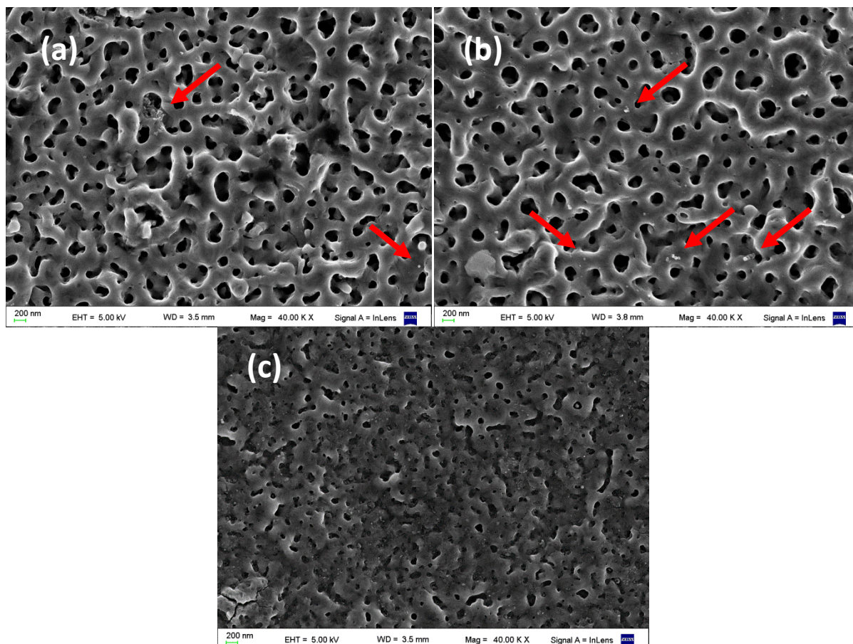
Figura 3.56: Micrografías electrónicas. Influencia del Fe como dopante en el electrolito Probetas (a) S4-V120-J1200-t5- Fe1 , (b) S4-V120-J1200-t2,5- Fe2 y (c) S4-V120-J1200-t1- Fe3 .
