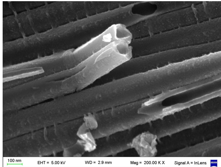
Figura 5.4: Micrografías electrónicas. Estrías en la pared de los NTL. Probeta EG-V60-t2.
