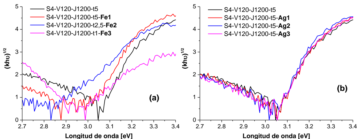
Figura 3.59: Gráficas Tauc. Influencia de dopantes en electrolito. Probetas (a) S4-V120-J1200-t5-Fe1, S4-V120-J1200-t2,5-Fe2 y S4-V120-J1200-t1-Fe3 y (b) S4-V120-J1200-t5-Ag1, S4-V120-J1200-t5-Ag2 y S4-V120-J1200-t5-Ag3.
