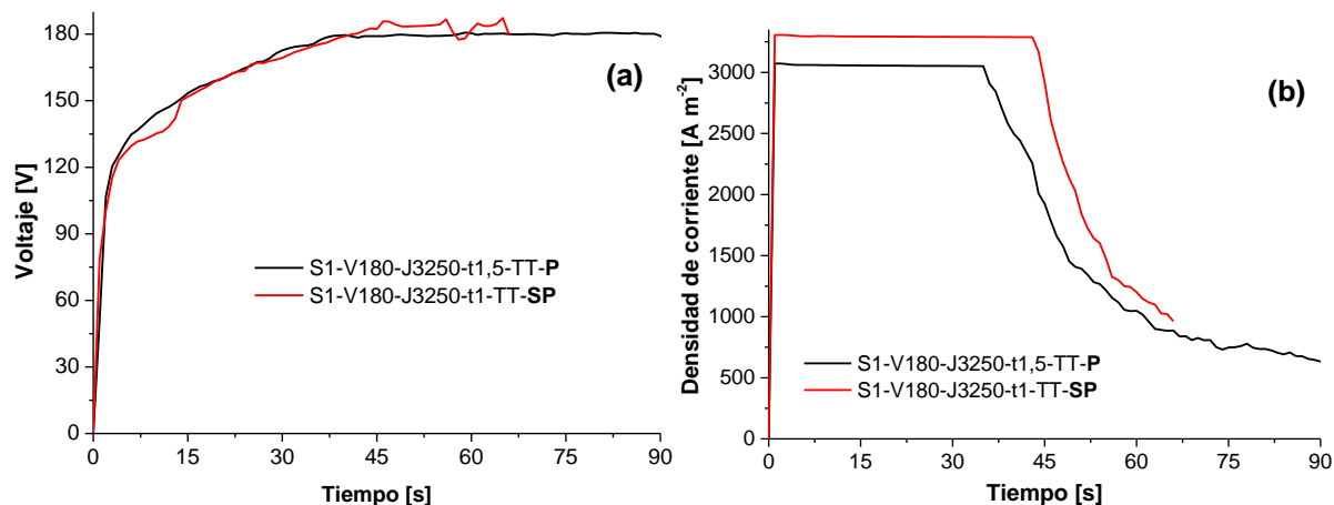
Figura I.2: Evolución temporal de (a) voltaje y (b) densidad de corriente. Influencia de la preparación superficial. Probetas S1-V180-J3250-t1,5-TT-P, S1-V180-J3250-t1-TT-SP.
