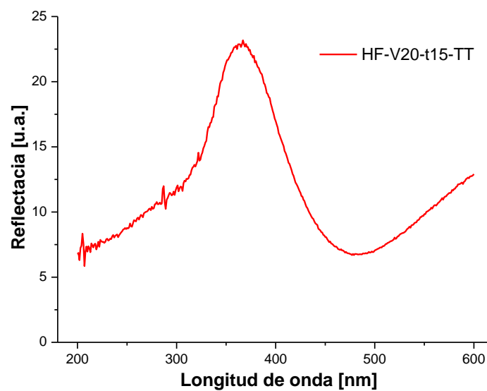
Figura 4.10: Espectro de reflectancia difusa de un recubrimiento NTC. Probeta HF-V20-t15-TT
