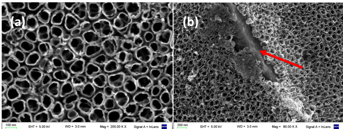
Figura 4.4: Micrografías electrónicas de recubrimientos NTC. Probeta HF-V20-t5-TT. (a) NTC, vista superior y (b) Influencia de acabado metalográfico. Flecha roja: raya del desbaste.
