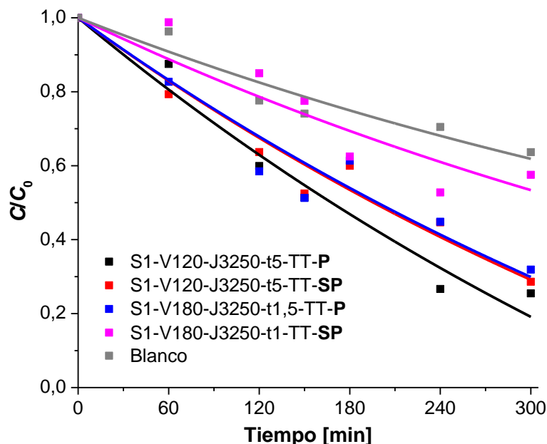
Figura I.7: Perfiles temporales de concentración normalizada de Cr(VI) ( C/C_0 ) para la reacción fotocatalítica en presencia de EDTA con las probetas S1-V120-J3250-t5-TT-P, S1-V120-J3250-t5-TT-SP, S1-V180-J3250-t1,5-TT-P, S1-V180-J3250-t1-TT-SP. Condiciones experimentales: [K_2Cr_2O_7] = 0,4 \text{ mM} , [EDTA] = 1 \text{ mM} , \text{pH } 2 , E_{365\text{nm}} = 2450 \mu\text{W}/\text{cm}^2 , T = 25 \text{ }^\circ\text{C} . Las líneas representan el ajuste de las curvas con la ecuación 3.4.
