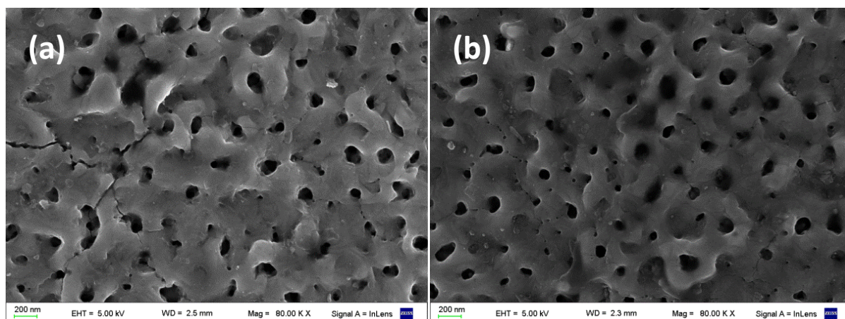
Figura I.3: Micrografías electrónicas. Influencia de la preparación superficial. Probetas (a) S1-V120-J3250-t5-TT-P (b) S1-V120-J3250-TT-SP.
