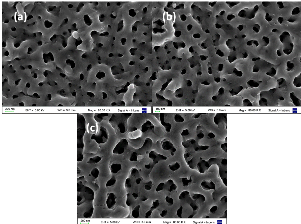
Figura 3.50: Micrografías electrónicas. Influencia del tiempo de anodización. Probetas (a) S4-V120-J1200-t05-TT, (b) S4-V120-J1200-t15-TT y (c) S4-V120-J1200-t60-TT.
