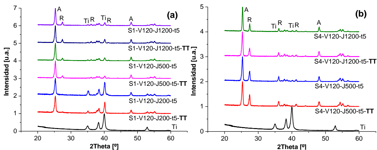
Figura III.2: Difractogramas normalizados. Influencia del tratamiento térmico. Sustrato (Ti) y probetas con y sin TT, anodizadas en H 2 SO 4 (a) 1 M y (b) 4 M.
