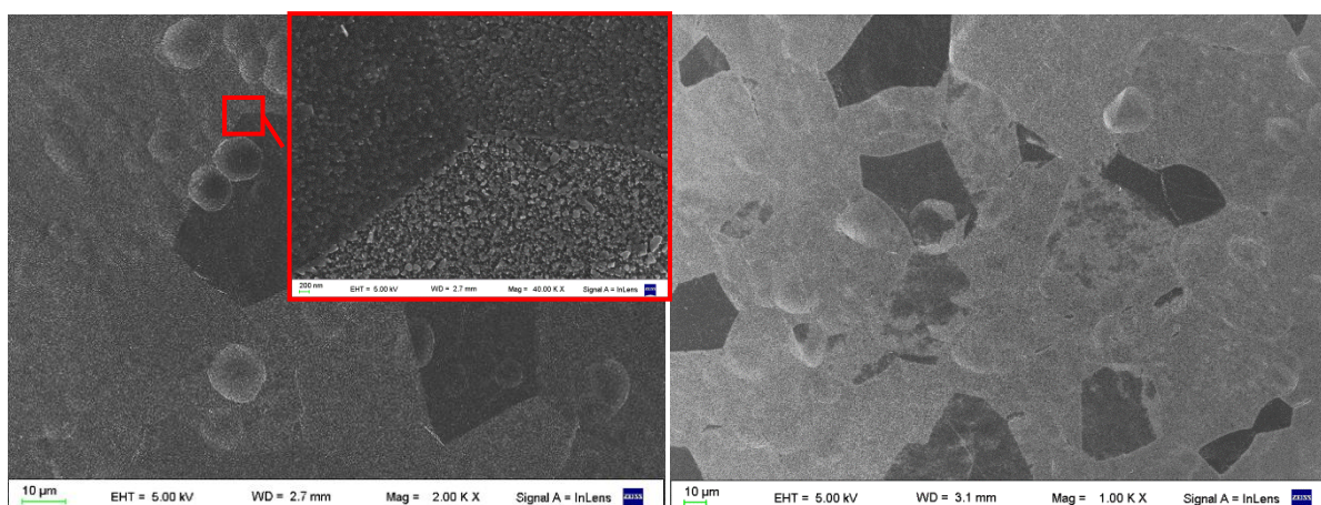
Figura 4.18: Micrográficas electrónicas. Influencia de la textura del sustrato. Probetas (a) HF-V20- t30 -TT, recubrimiento no nanotubular y (b) HF-V20- t120 -TT, recubrimiento nanotubular en “zonas claras”.
