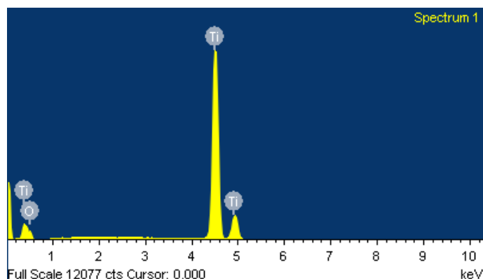
Figura 4.7: Análisis composicional. Recubrimiento NTC. Probeta HF-V20-t120-TT.
