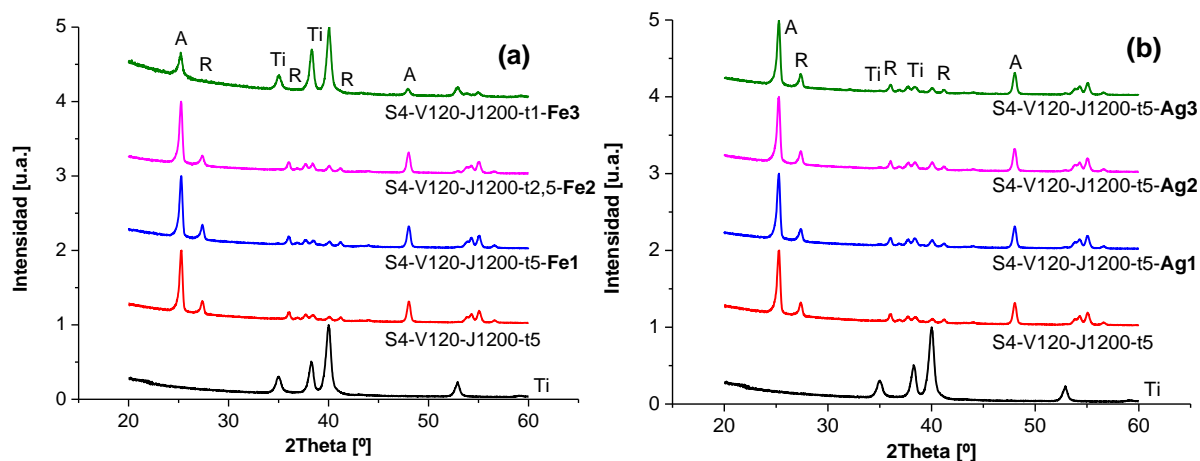
Figura 3.58: Difractogramas normalizados. Influencia de dopantes en el electrolito. Sustrato (Ti), una probeta de referencia y las probetas (a) S4-V120-J1200-t5-Fe1, S4-V120-J1200-t2,5-Fe2 y S4-V120-J1200-t1-Fe3 y (b) S4-V120-J1200-t5-Ag1, S4-V120-J1200-t5-Ag2 y S4-V120-J1200-t5-Ag3. A: anatasa; R: rutilo; Ti: titanio.
