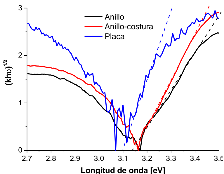
Figura 6.17: Gráficas Tauc. Evaluación de la geometría del sustrato: placas, anillo, zona de costura y anillo, zona sin costura.
