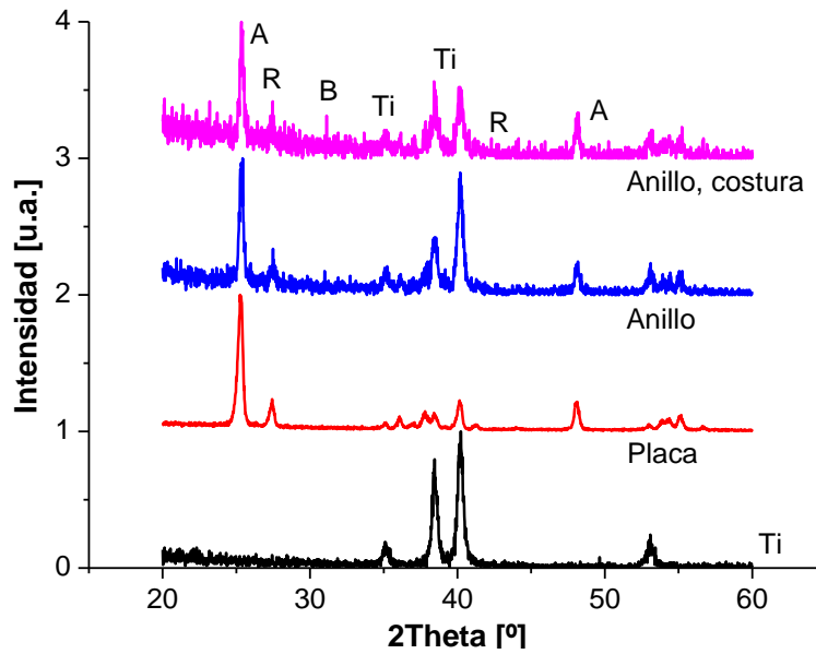
Figura 6.15: Difractogramas normalizados. Evaluación de la geometría del sustrato y costura. Condiciones de anodización: S1-V120-J1200-t5-TT.
