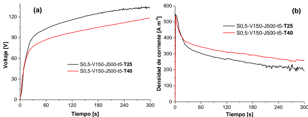
Figura II.1: Evolución temporal de (a) voltaje y (b) densidad de corriente. Influencia de la temperatura del electrolito. Probetas S0,5-V150-J500-t5-T25 y S0,5-V150-J500-t5-T40.
