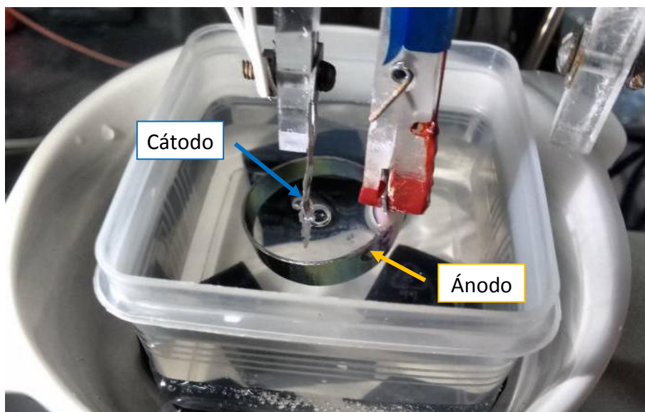
Figura 6.5: Fotografía de la configuración de la celda electroquímica durante la anodización de anillos. Cátodo ubicado en el centro del anillo (ánodo).
