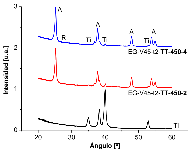
Figura 5.20: Difractogramas normalizados. Influencia del tiempo de TT. Sustrato (Ti) y probetas EG-V45-t2-TT-450-2 y EG-V45-t2-TT-450-4.
