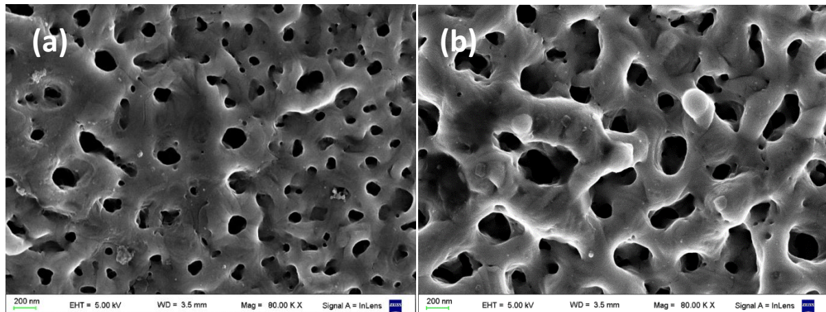
Figura 3.33: Micrografías electrónicas. Influencia de la concentración del electrolito. Probetas (a) S1-V120-J500-t5-TT y (b) S4-V120-J500-t5-TT .
