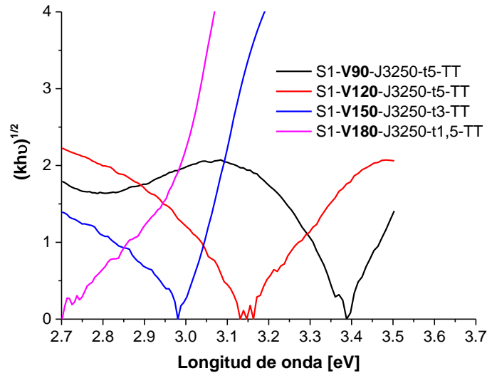
Figura 3.29: Gráficas Tauc. Influencia del voltaje. Probetas Probetas S1-V90-J3250-t5-TT, S1-V120-J3250-t5-TT, S1-V150-J3250-t3-TT y S1-V180-J3250-t1,5-TT.
