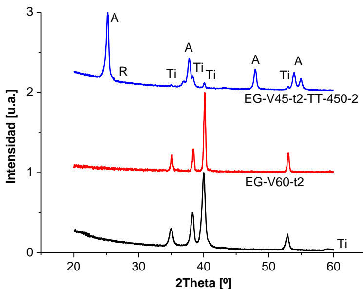
Figura 5.5: Difractogramas normalizados. Sustrato (Ti) y probetas EG-V60-t2 y EG-V45-t2-TT-450-2. A: anatasa; R: rutilo; Ti: titanio.
