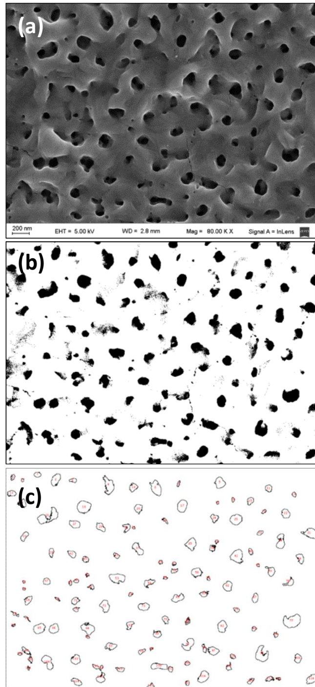
Figura 3.10: Etapas del procesamiento de imágenes realizado en ImageJ. (a) Micrografía original (b) Micrografía sin rótulo y binarizada y (c) Distinción de los poros por análisis de partículas.
