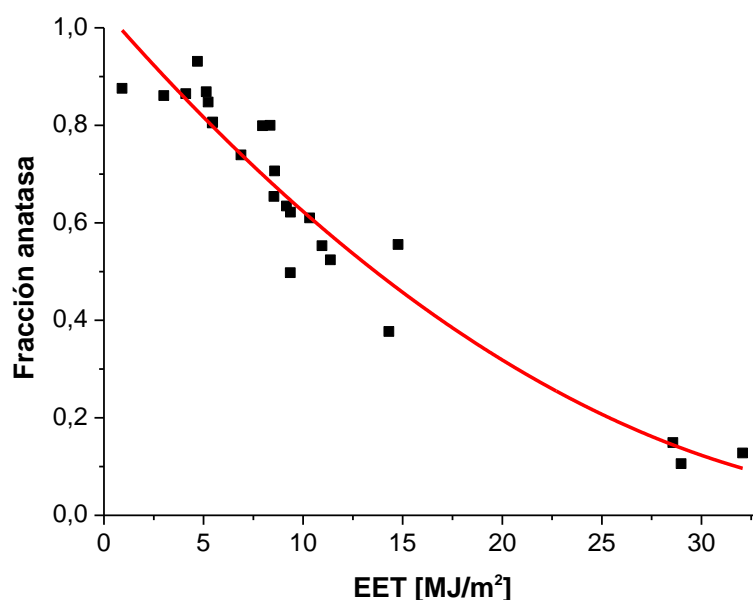
Figura 3.63: Fracción anatasa vs. energía específica total ( EET ). Puntos experimentales y ajuste con ecuación polinómica segundo orden del tipo y = a*x^2 + b*x + c .
