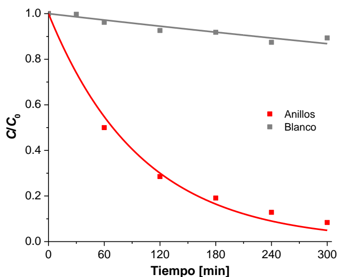
Figura 6.18: Perfiles temporales de concentración normalizada de Cr(VI) ( C/C_0 ) para la reacción fotocatalítica de reducción de Cr(VI) en presencia de EDTA en el reactor anular empleando anillos recubiertos de \text{TiO}_2 . Condiciones experimentales: [\text{K}_2\text{Cr}_2\text{O}_7] = 0,4 \text{ mM} , [\text{EDTA}] = 1 \text{ mM} , \text{pH } 2 , E_{365\text{nm}} = 2800 \mu\text{W}/\text{cm}^2 , T = 25 \text{ }^\circ\text{C} . Las líneas representan el ajuste de las curvas con la ecuación 3.4.
