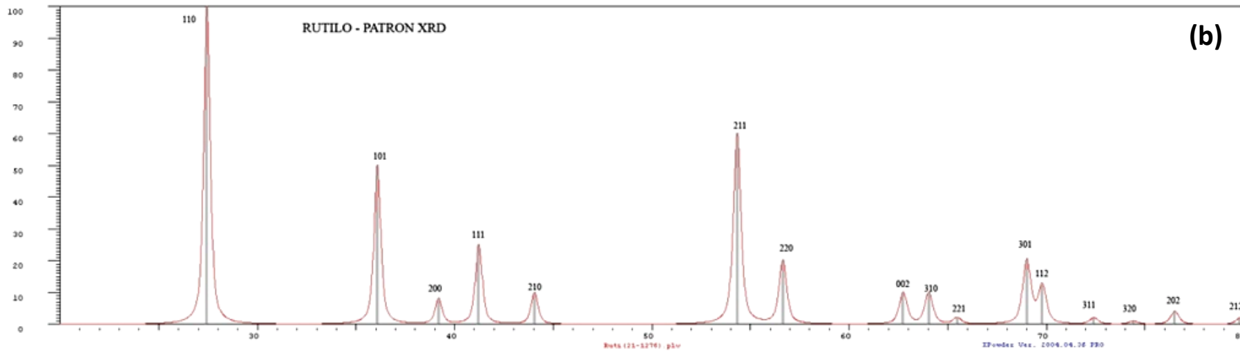
Figura 2.8: Espectros característicos de \text{TiO}_2 . (a) anatasa y (b) rutilo. Adaptado de [121,122]
