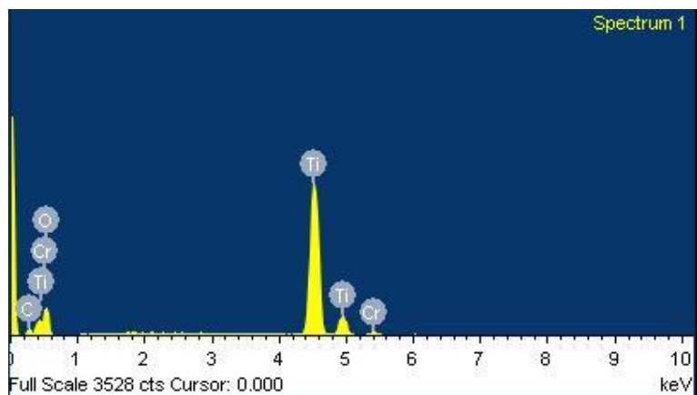
Figura 5.6: Análisis composicional de un recubrimiento. Probeta EG-V40-t5-TT-450-2
