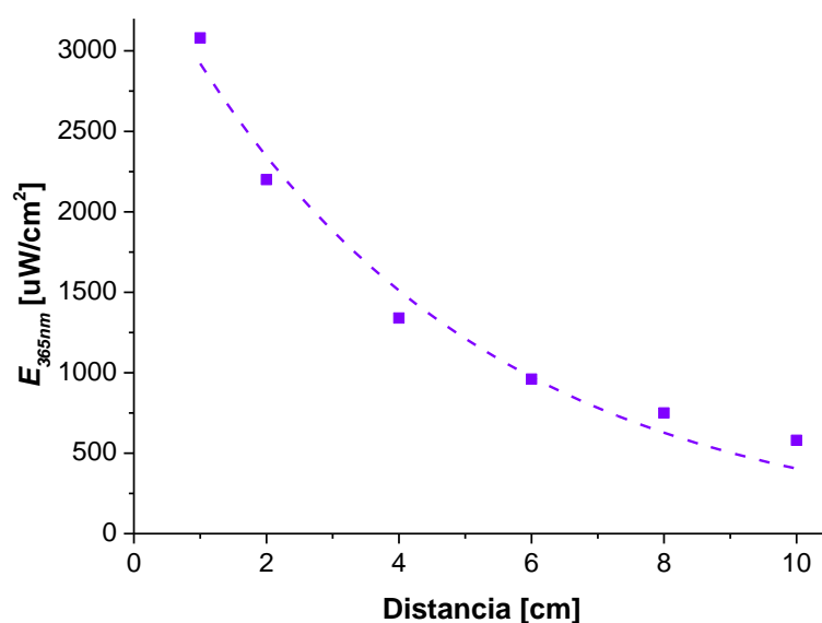
Figura 6.12: Variación de la irradiancia a 365 nm de la lámpara del fotorreactor en función de la distancia entre la fuente de luz y el radiómetro.
