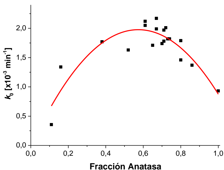
Figura 3.62: Fracción anatasa vs. constante cinética de orden cero ( k_0 ). Puntos experimentales y ajuste con ecuación polinómica segundo orden del tipo y = a \cdot x^2 + b \cdot x + c .
