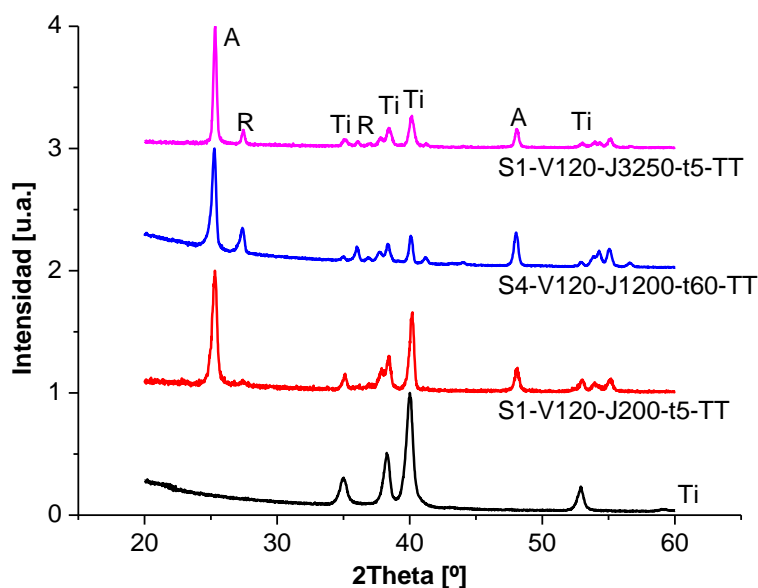
Figura 3.21: Difractogramas normalizados. Sustrato (Ti) y probetas S1-V120-J200-t5-TT, S4-V120-J1200-t60-TT y S1-V120-J3250-t5-TT. A: anatasa; R: rutilo; Ti: titanio.
