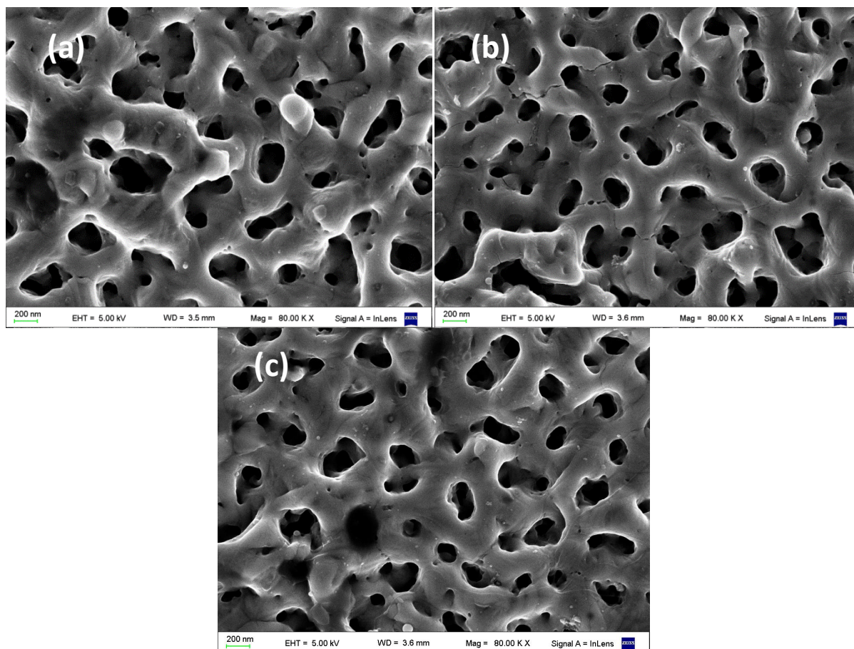
Figura 3.44: Micrografías electrónicas. Influencia de la densidad de corriente. Probetas (a) S4-V120-J500-t5-TT , (b) S4-V120-J1200-t5-TT y (c) S4-V120-J3000-t3-TT .
