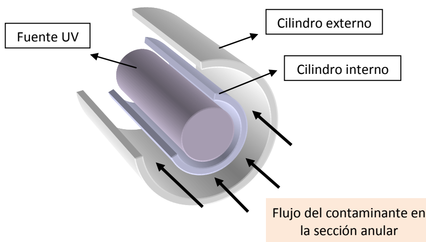
Figura 6.6: Representación de un reactor anular concéntrico con fuente de luz en el centro. Las flechas indican sentido del flujo del contaminante por la sección anular.
