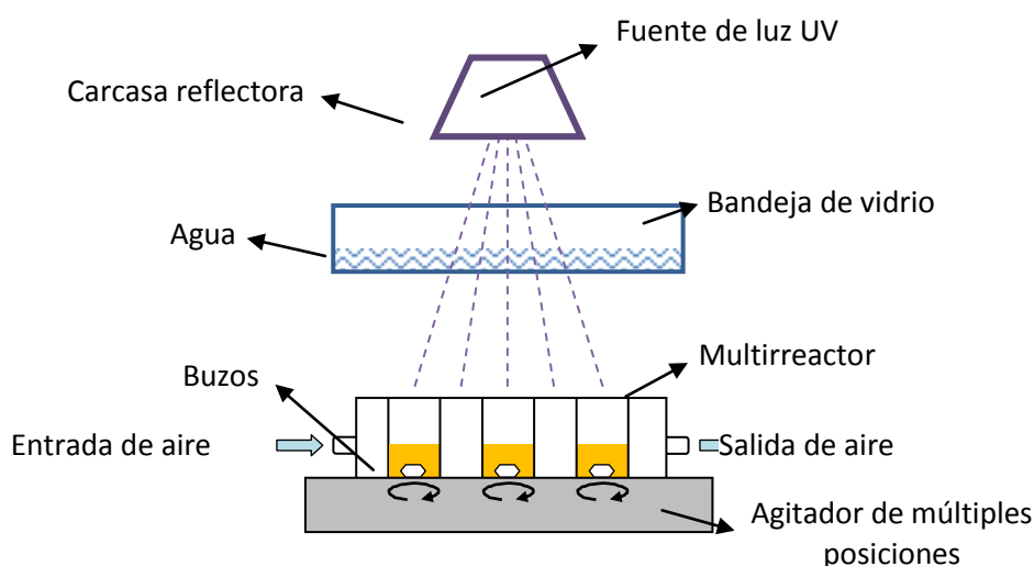
Figura 3.14: Esquema del arreglo experimental para los experimentos fotocatalíticos.
