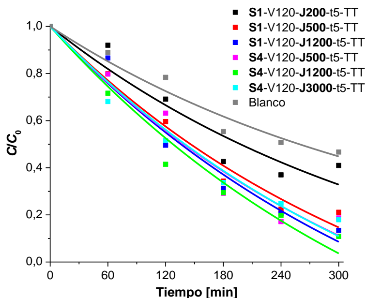
Figura 3.47: Perfiles temporales de concentración normalizada de Cr(VI) ( C/C_0 ) para la reacción fotocatalítica en presencia de EDTA con las probetas S1-V120-J200-t5-TT , S1-V120-J500-t5-TT , S1-V120-J1200-t5-TT , S4-V120-J500-t5-TT , S4-V120-J1200-t5-TT y S4-V120-J3000-t3-TT . Condiciones experimentales: [K_2Cr_2O_7] = 0,4 \text{ mM} , [EDTA] = 1 \text{ mM} , \text{pH } 2 , E_{365\text{nm}} = 3700 \text{ } \mu\text{W}/\text{cm}^2 , T = 25 \text{ } ^\circ\text{C} . Las líneas representan el ajuste de las curvas con la ecuación 3.4.
