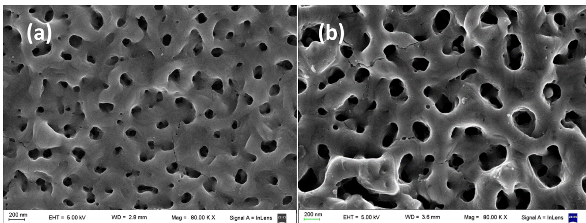
Figura 3.34: Micrografías electrónicas. Influencia de la concentración del electrolito. Probetas (a) S1-V120-J1200-t5-TT y (b) S4-V120-J1200-t5-TT .
