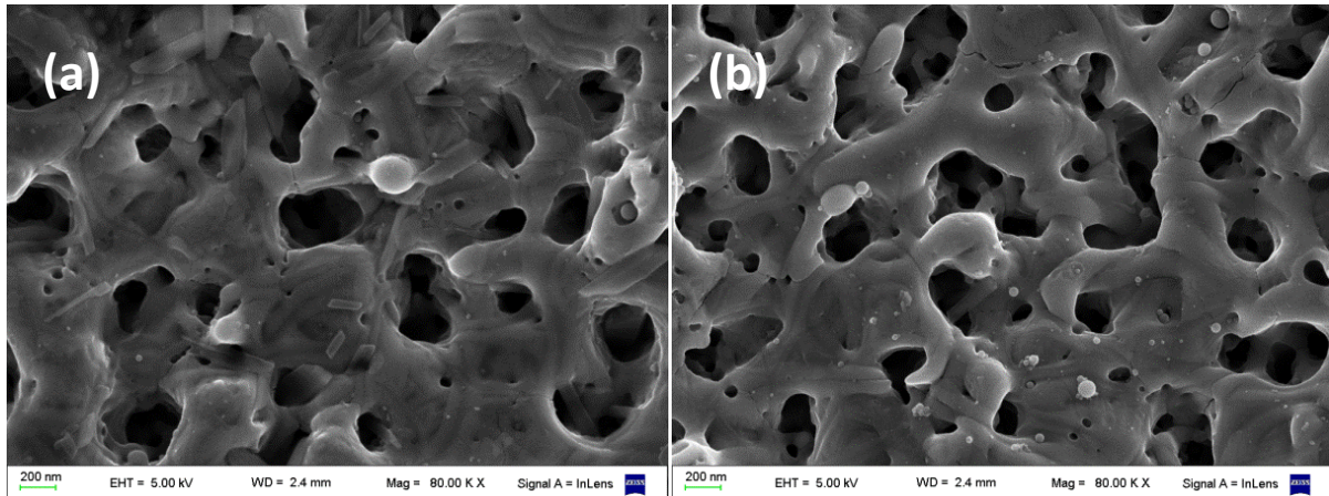
Figura I.4: Micrografías electrónicas. Influencia de la preparación superficial. Probetas (a) S1-V180-J3250-t1,5-TT-P (b) S1-V180-J3250-t1- TT-SP.
