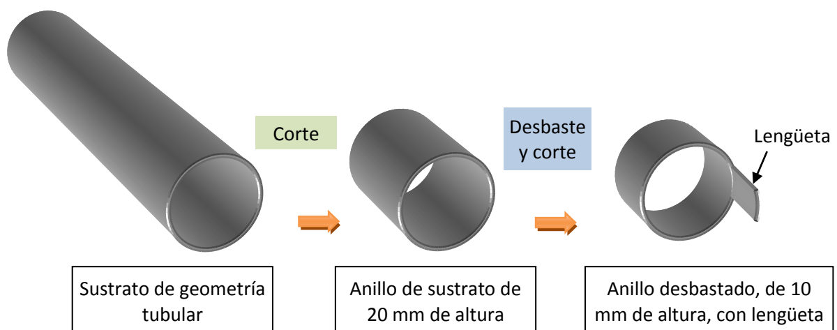
Figura 6.3: Secuencia de cortes y desbaste del sustrato tubular.
