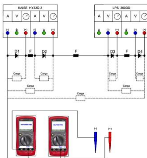
Figura 3.5: Diagrama de conexiones de equipo de oxidación anódica.
