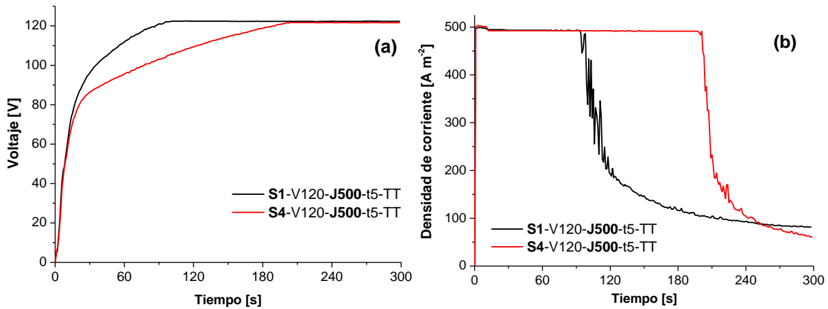
Figura 3.31: Evolución temporal del (a) voltaje y (b) la densidad de corriente. Influencia de la concentración del electrolito. Probetas S1-V120-J500-t5-TT , S4-V120-J500-t5-TT .
