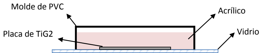
Figura 3.2: Diagrama del método de inclusión de probetas rectangulares.
