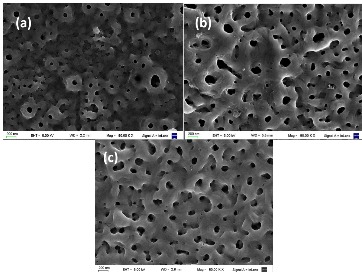
Figura 3.43: Micrografías electrónicas. Influencia de la densidad de corriente. Probetas (a) S1-V120-J200-t5-TT , (b) S1-V120-J500-t5-TT y (c) S1-V120-J1200-t5-TT .
