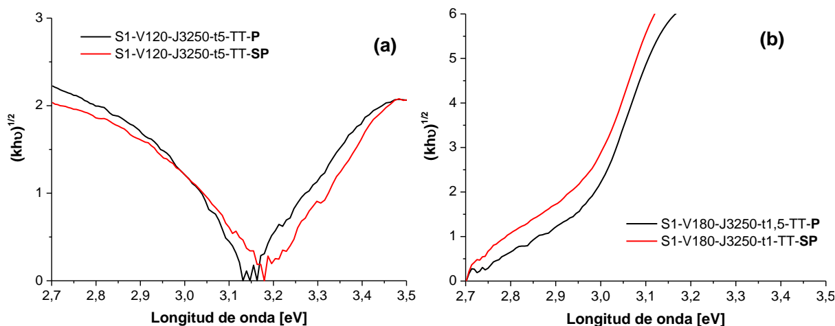
Figura I.6: Gráficas Tauc. Influencia de la preparación superficial. Probetas (a) S1-V120-J3250-t5-TT-P y S1-V120-J3250-t5-TT-SP y (b) S1-V180-J3250-t1,5-TT-P, S1-V180-J3250-t1-TT-SP.
