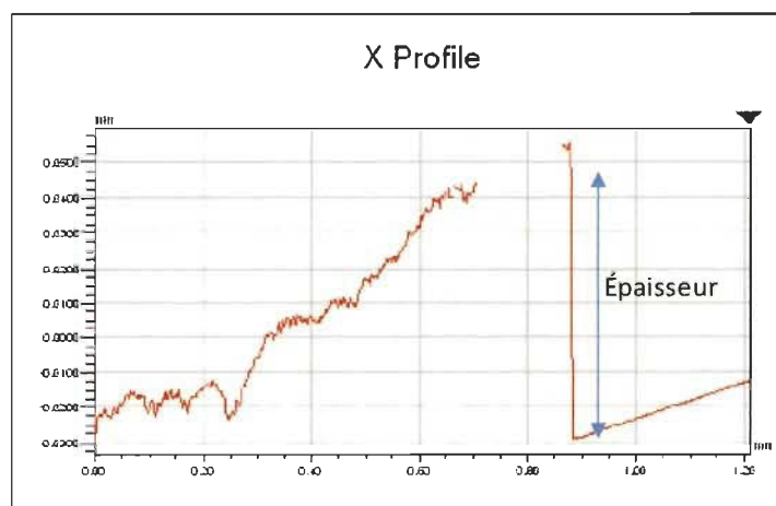
Figure 4.15 : Mesure de l'épaisseur de la membrane
