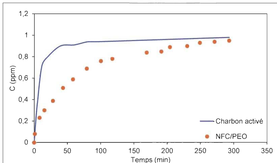
Figure 4.37 : Comparaison entre le charbon activé et les NFC/PEO dans les mêmes conditions d'écoulement et de concentration (1 ppm et 10 ml/min)
