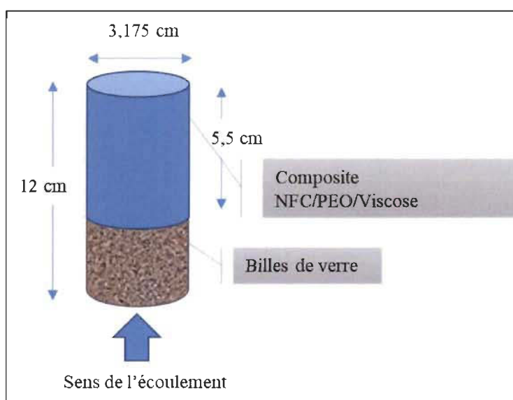
Figure 3.6 : Dimensions de la colonne d'adsorption
