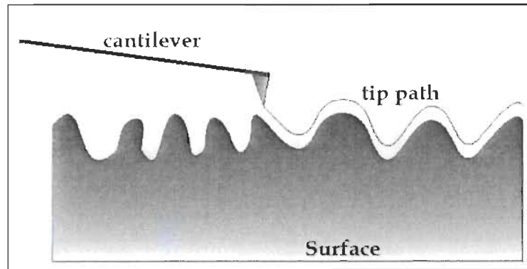
Figure 2.12: Principe de fonctionnement de l'AFM (De Oliveira, Albuquerque [47])
