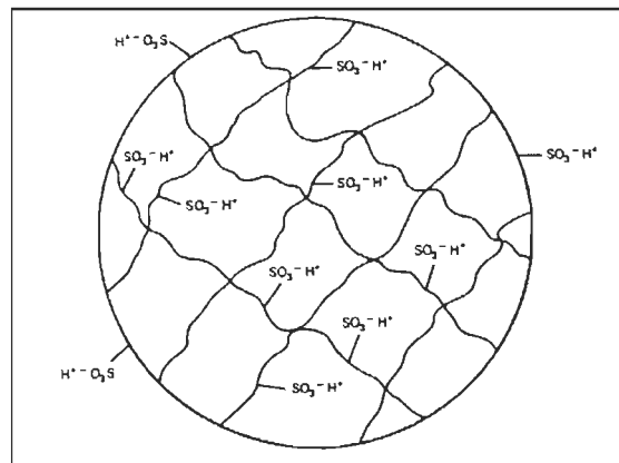
Figure 2.2 : Schéma de la résine échangeuse de cations montrant la matrice chargée négativement et les ions positifs échangeables (R. M. Wheaton [15])
