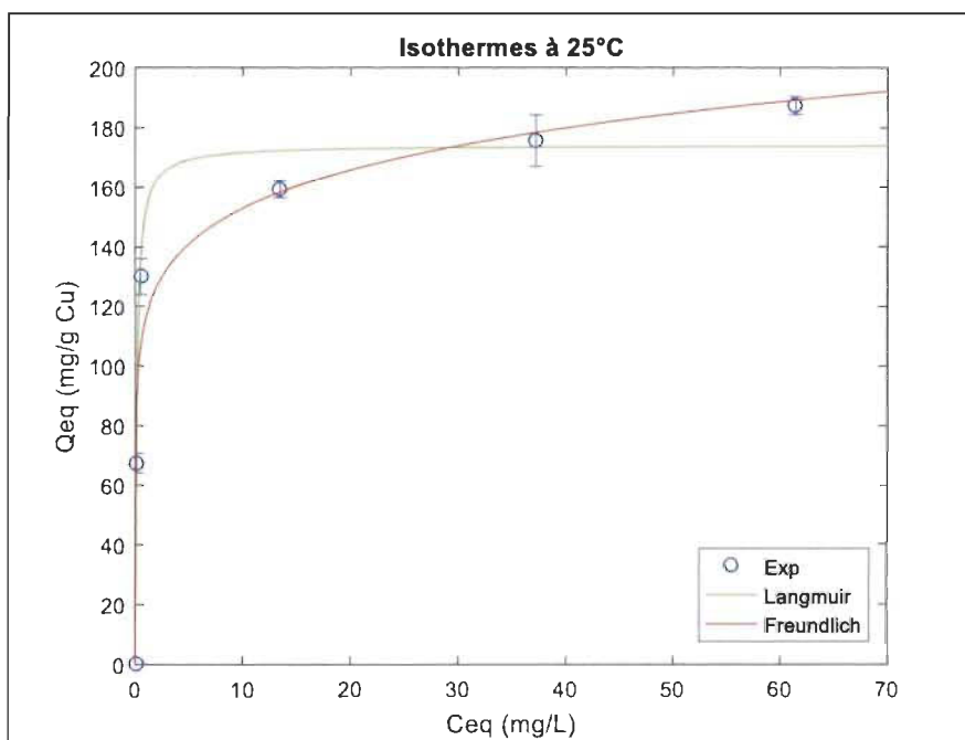
Figure 4.17 : Isothermes d'adsorption du cuivre à 25°C pour les membranes préparées
