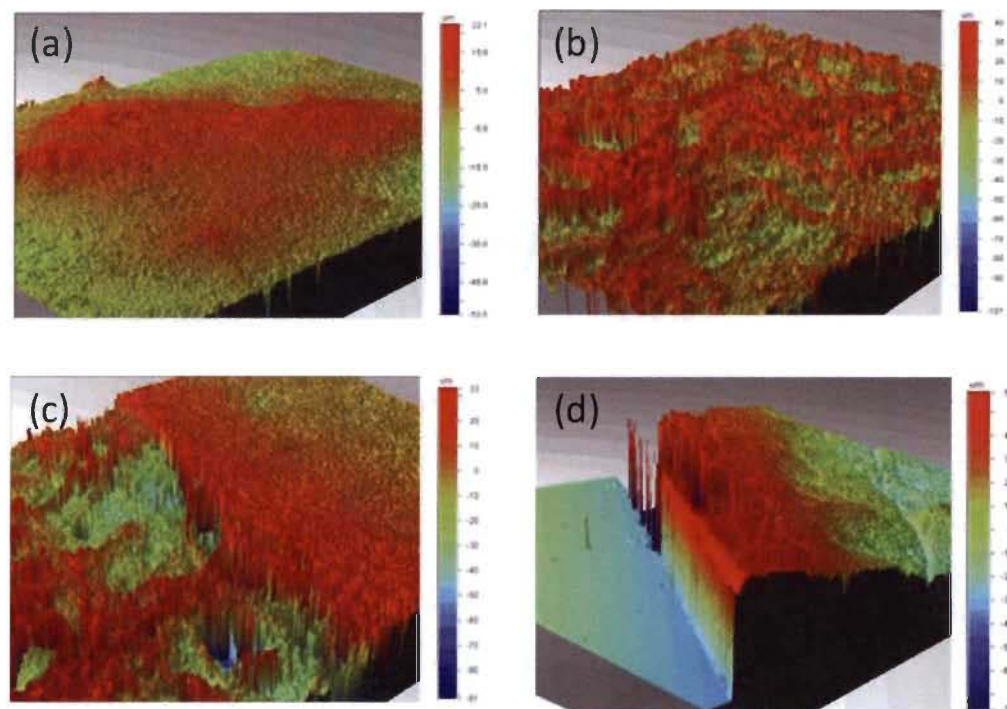
Figure 4.14 : Profil de la membrane NFC/PEO (a), Profil du support (b), différence de rugosité entre la membrane et le support (c), épaisseur en 3D (d)
