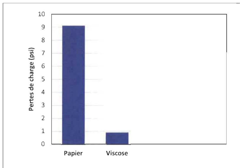
Figure 4.4 : Pertes de charges pour un empilement de 4 couches de support
