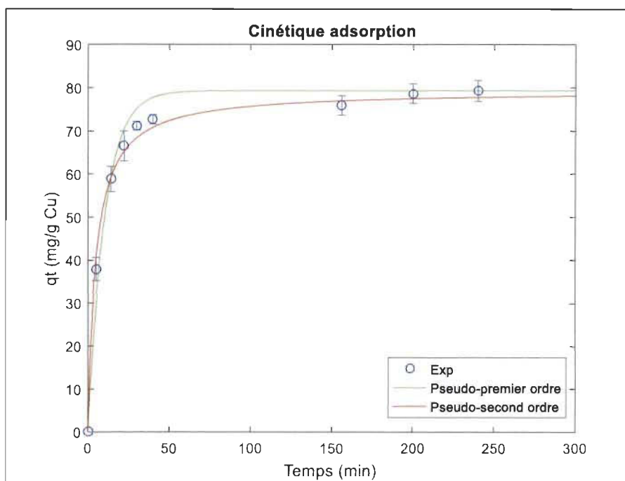
Figure 4.18 : Courbe expérimentale de cinétique d'adsorption et corrélation avec les modèles de cinétique de réaction
