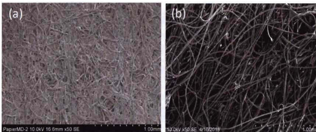
Figure 4.5 : Images MEB; (a) des fibres de papier, (b) des fibres de viscose
