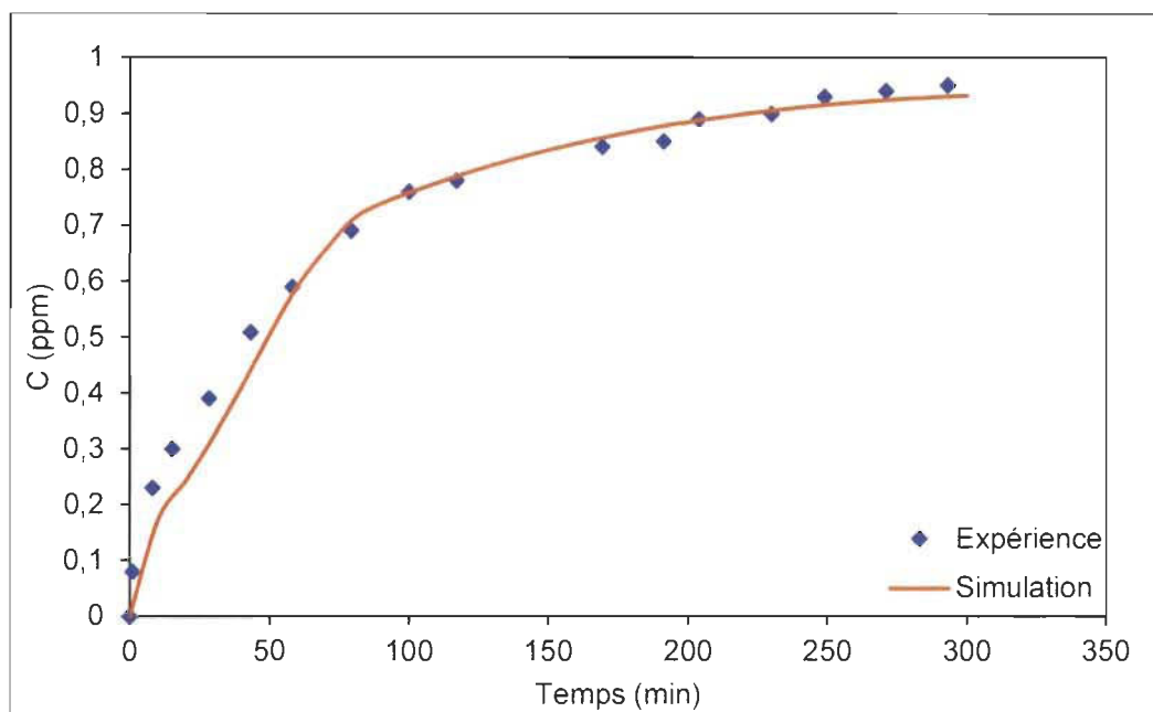
Figure 4.31 : Comparaison des résultats expérimentaux avec ceux de la simulation pour une concentration de 1 ppm et un débit de 10 mL/min
