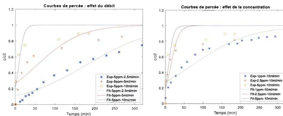
Figure 4.25 : Corrélation des courbes de percée par le modèle de Thomas (Équation 2.14)
