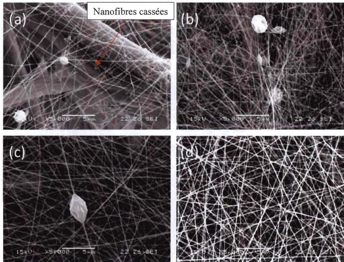
Figure 4.10 : Image MEB des membranes de NFC en fonction du temps d'électrofilage; (a) 30 min, (b) 1 heure, (c) 2 heures et (d) 3 heures pour la même distance injecteur-collecteur.
