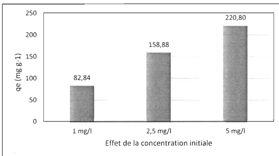
Figure 4.23 : Effet de la variation de la concentration initiale sur la capacité d'adsorption
