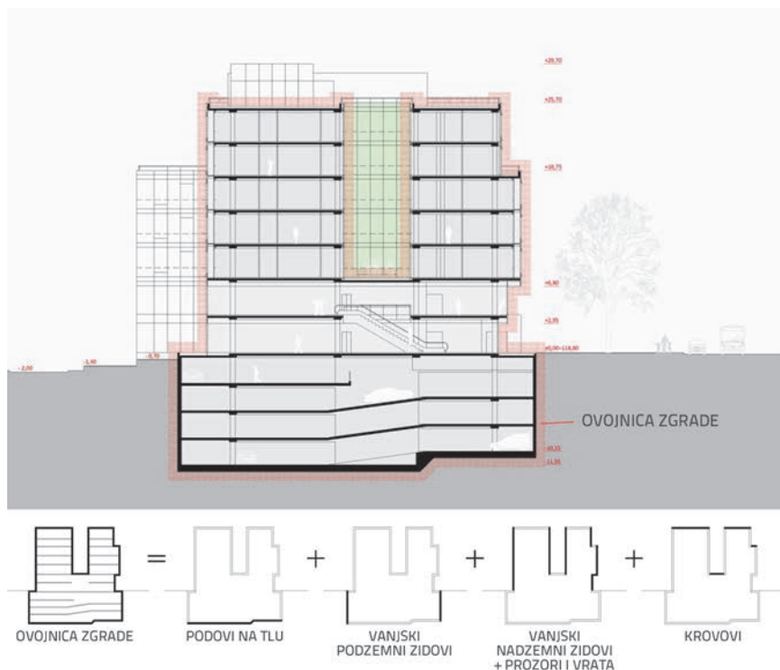
Slika 3. Ovojnica zgrade
