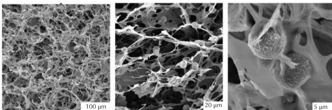
Slika 14 – SEM mikrografije osušenog hidrogela s HAp česticama precipitiranim in situ unutar kitozanske matrice 28
