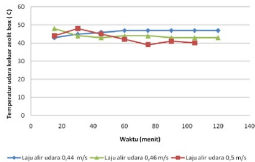
Gambar 2. Temperatur udara keluar ruang pengering
