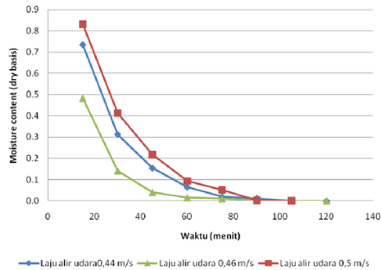
Gambar 5. Grafik hubungan antara kadar air dan waktu.
