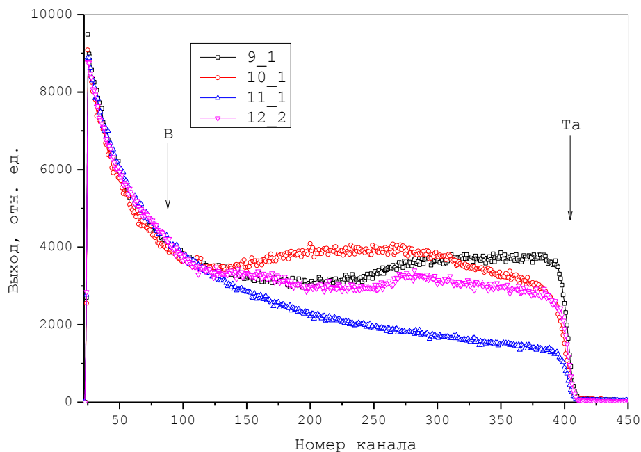
Рисунок 8. Спектри POP для чотирьох зразків з покриттями \text{TaV}_2 .
