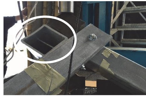
(d) Deformed profile
