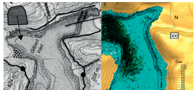
Figura 18. Comparación de los datos de Fritz[35] (izquierda) con los resultados del cálculo (derecha; curvas de nivel cada 100 m). Se muestra una superposición de imágenes de los resultados en distintos pasos de tiempo.
