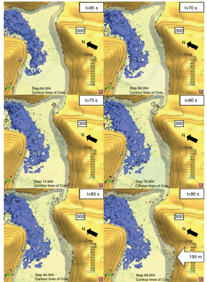
Figura 17. Propagación de la ola en la bahía y alcance máximo en la margen sur. Curvas de nivel cada 100 m.
