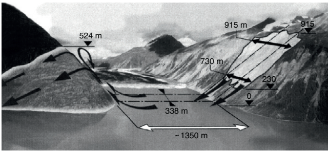
Figura 14. Esquema del deslizamiento de Lituya Bay. La destrucción del bosque de la ladera izquierda corresponde con la cota alcanzada por la ola generada (Fritz et al. [35]).
