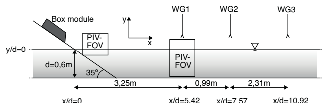
Figura 10. Esquema del experimento de Sælevik et al. [13], con la situación de los sensores.
