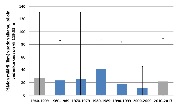
Kuva 5.7. Päivien määrä vuoden aikana, jolloin vedenkorkeus on ollut yli N_{\text{hanke}} + 119,35 m. Pylvään korkeus esittää mittarin keskimääräisen arvon ja jana vaihteluvälin esitettyltä jaksolta. Vertailujakso ja viimeisten kahdeksan vuoden tarkastelujakso ovat harmaalla.
