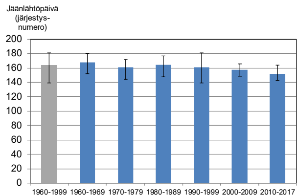
Kuva 4.11. Inarijärven selkavesien jäänlähtö eri tarkastelujaksosilla. Pylvään korkeus esittää mittarin keskimääräisen arvon ja jana todellisen vaihteluvälin tarkastelujaksolla.
