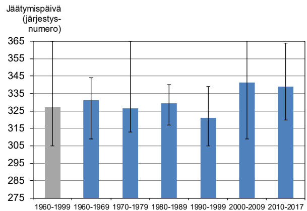
Kuva 4.10. Inarijärven selkavesien jätymisen eri tarkastelujaksosilla. Pylvään korkeus esittää mittarin keskimääräisen arvon ja jana todellisen vaihteluvälin tarkastelujaksolla. Vuonna 2006 jätymispäivä oli vasta seuraavana vuonna, jolloin jakson 2000–2009 maksimi on suurempi kuin 365.
