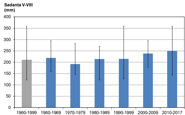
Kuva 4.3. Touko-elokuun sadanta eri tarkastelujaksoilla. Pylvään korkeus esittää mittarin keskimääräisen arvon ja jana todellisen vaihteluvälin tarkastelujaksolla.
