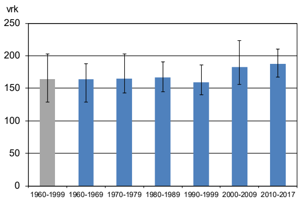
Kuva 4.12. Avovesikauden pituus Inarijärven eri tarkastelujaksosilla. Pylvään korkeus esittää mittarin keskimääräisen arvon ja jana todellisen vaihteluvälin tarkastelujaksolla.
