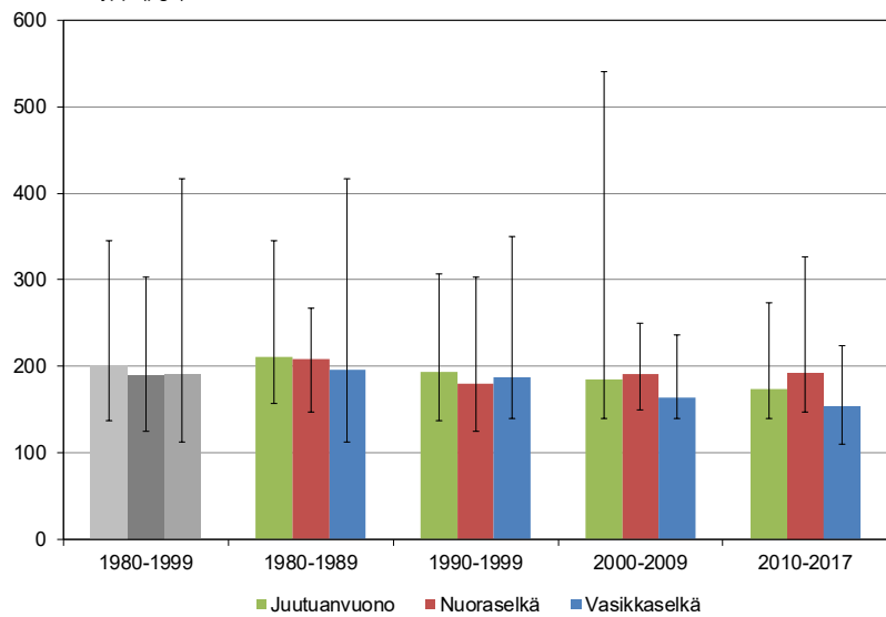
Kuva 6.10. Kokonaistyyppien keskipitoisuus Juutuanvuonon, Nuoraselän ja Vasikkaselän havaintopaikoilla eri tarkastelujaksolla. Pylvään korkeus esittää mittarin keskimääräisen arvon ja jana vaihteluvälin tarkastelujaksolla.
