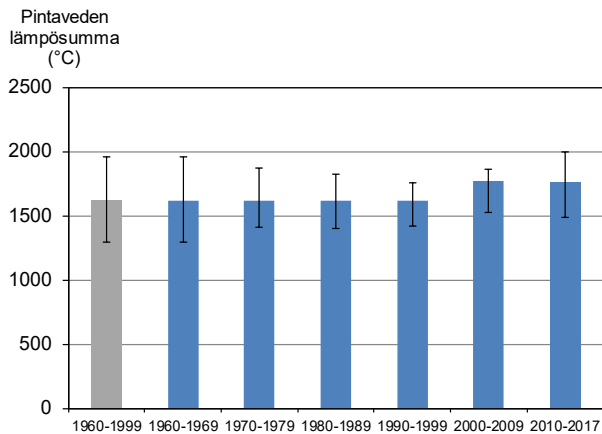
Kuva 4.8. Avovesikauden lämpösumma eri tarkastelujaksoilla. Pylvään korkeus esittää mittarin keskimääräisen arvon ja jana todellisen vaihteluvälin tarkastelujaksolla.
