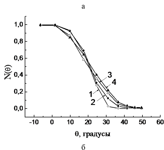
Рисунок 2 – Корректирующие коэффициенты (а) и нормированный сигнал камеры N(\theta) (б) в зависимости от положения сканирующего отверстия для пленок лавсана различной плотности, \text{г/м}^2 . а: 1 – 0; 2 – 69; 3 – 178; 4 – 400. б: 1 – \xi_1 ; 2 – \xi_2
