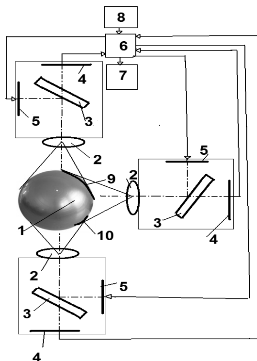
Рисунок 5 – Устройство для инфракрасного нагрева
