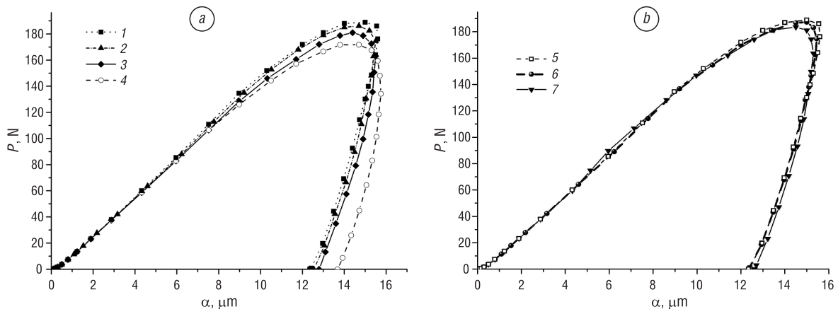
Рис. 5. Типичные диаграммы контактное усилие – перемещение при индентировании пластины твердостью 105 НВ ( \sigma_0 = 200 МПа), толщиной 5 мм ( a ) и 12 мм ( b ): 1, 5 – внедрение в полупространство материала (жесткая пластина); расстояние от места заделки: 2, 6 – 5 мм, 3 – 10 мм, 4, 7 – 80 мм
