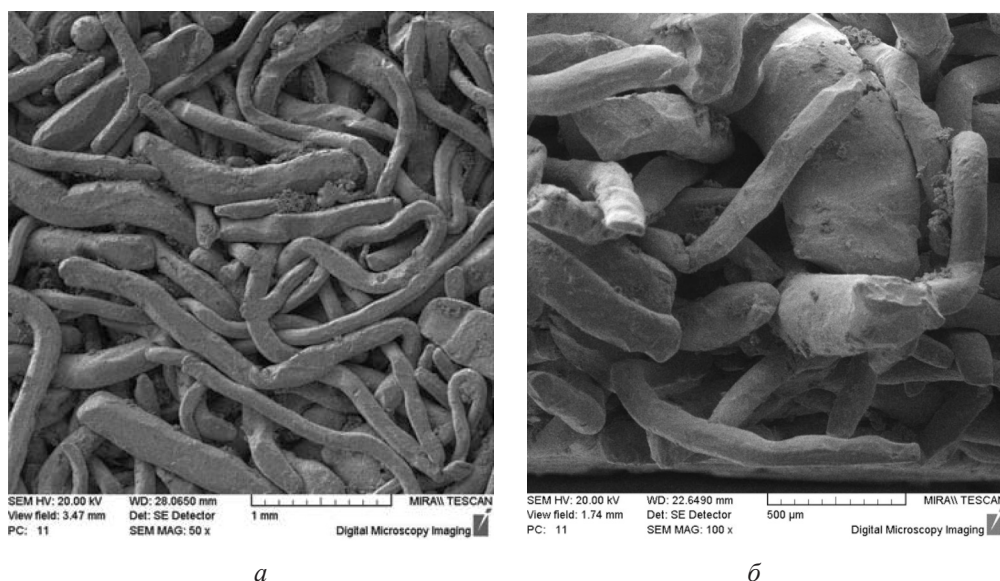
Рис. 2. Морфология поверхности (а) и излома спеченных при 1050 °С (б) образцов, изготовленных из дискретных медных волокон
