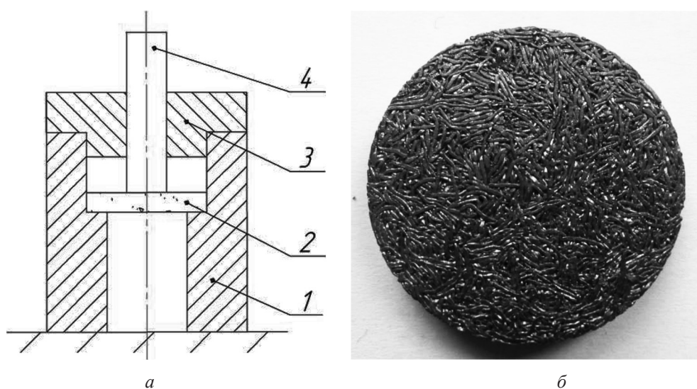
Рис. 1. Устройство для оценки качества спекания пористых волокновых материалов (а) и внешний вид образца для проведения испытаний (б)
