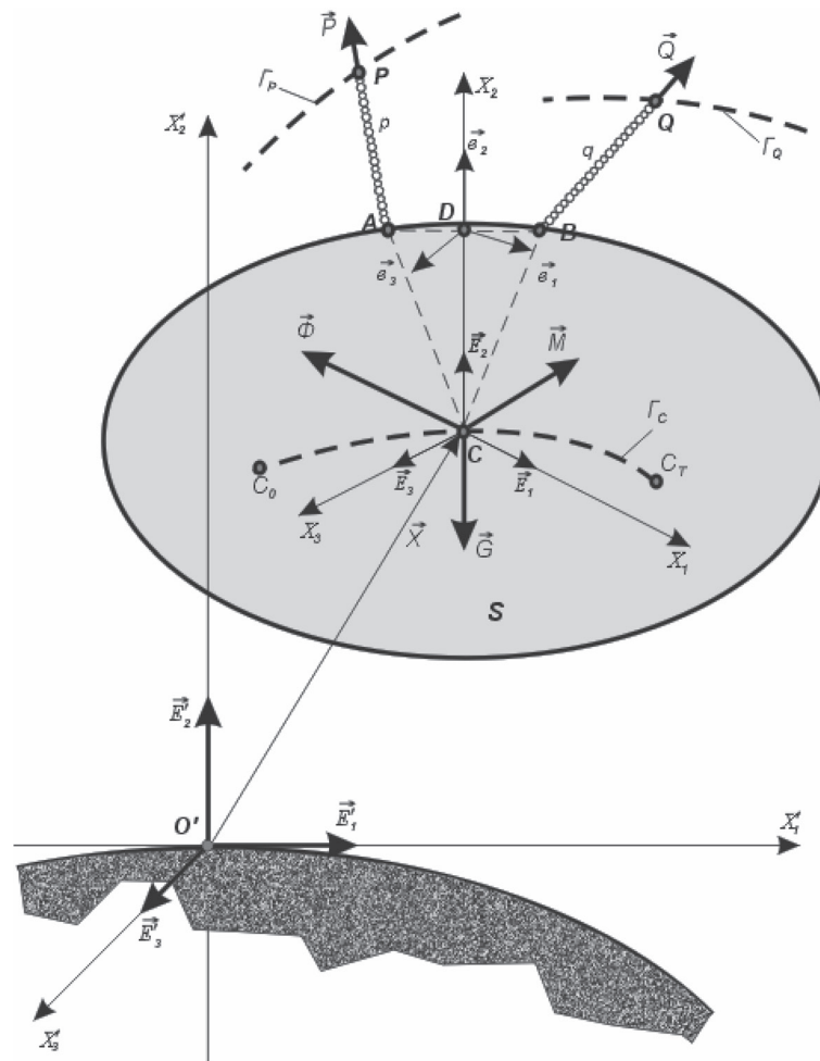
Кинетическая схема мобильного бифилярного подвеса тела S
