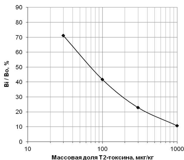
Рис. 3. Типичный градуировочный график набора реагентов ИФА-ТОКСИН Т-2
