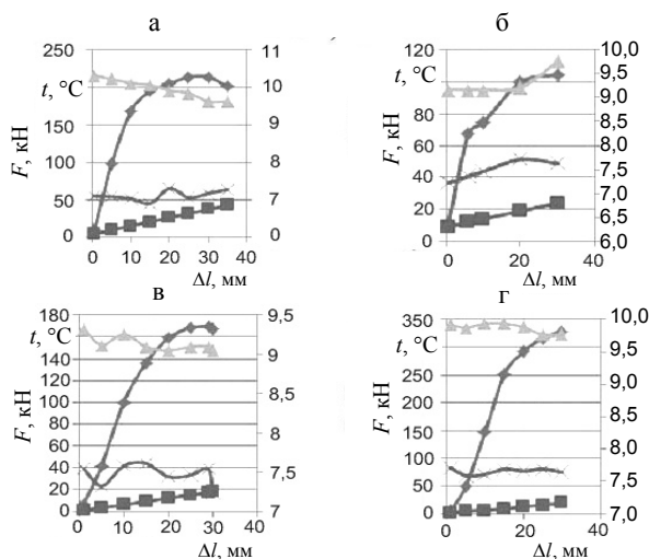
Рис. 5. Изменение наибольшей и наименьшей температур поверхности рабочей зоны образцов № 1 (а), 2 (б), 3 (в), 4 (г) при деформировании по возрастающей ветви диаграммы: ♦ – диаграммы растяжения образцов; ■ – кадры термофильма их деформирования; ▲ – температура поверхности образцов t_{max} , °С; × – то же t_{min} , °С
