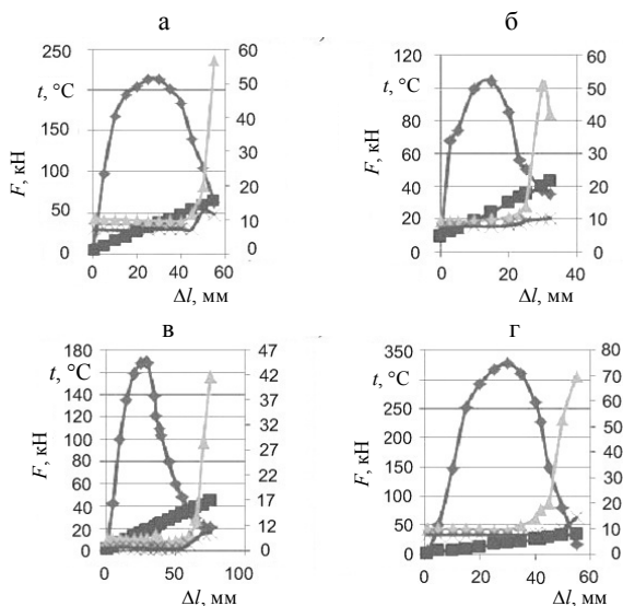
Рис. 4. Изменение наибольшей и наименьшей температур поверхности рабочей зоны образцов № 1 (а), 2 (б), 3 (в), 4 (г) при деформировании: ♦ – диаграммы растяжения образцов; ■ – кадры термофильма их деформирования; ▲ – температура поверхности образцов t_{max} , °С; × – то же t_{min} , °С
