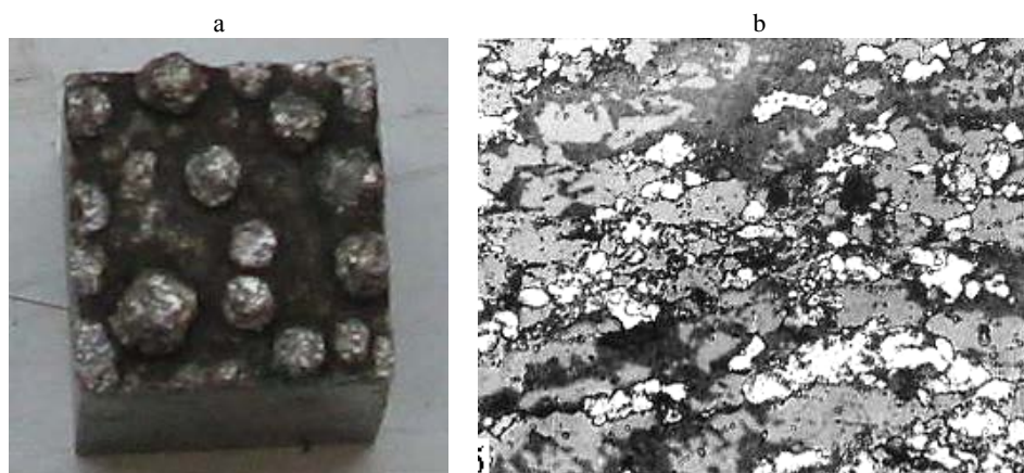
Рис. 2. Макро- (а) и микроструктура (b) сплава «колмоной» + 10 % WC», ×250 Fig. 2. Macro- (a) and microstructure (b) of “colmonoy” alloy + 10 % WC”, ×250
