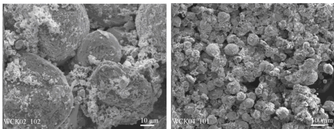
Рис. 1. Внешний вид композиции «колмоной» + 10 % WC» Fig. 1. External view of “colmonoy” composition + 10 % WC”
