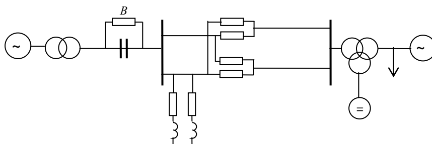
Рис. 3. Схема системы передачи с послеаварийной продольной компенсацией
