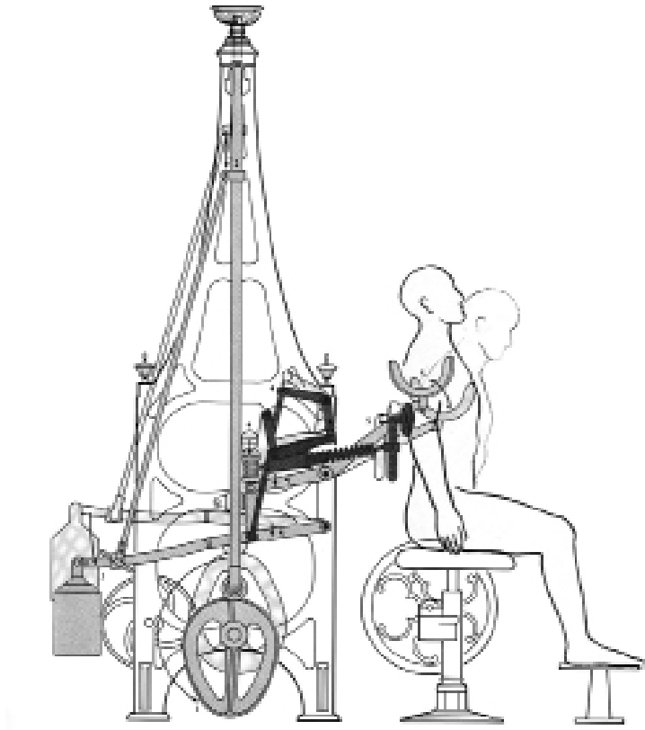
Figuur 4b: Dit toestel E6 wordt beschouwd als het "pièce de résistance" van de gehele collectie Zander apparaten in het Boerhaave Museum. Het is bedoeld om via passieve ademhaling de borstkas te verwijden en de bloedsomloop in de longen te bevorderen. Twee okselsteunen bewegen evenals een rugkussentje ritmisch op en neer, aangedreven door een drijfriem. De omvang van de beweging kon nauwkeurig ingesteld worden.(4)
