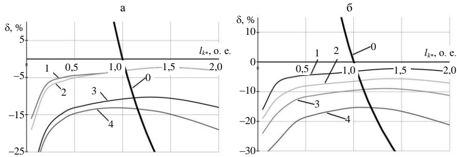
Рис. 3. Относительные погрешности определения l_{k^*} при различных видах КЗ и величинах нагрузки линии: 0 – кривая предельных погрешностей; а – 1 – при трехфазном КЗ и I_{нагр} = 0 ; 2 – при двухфазном КЗ и I_{нагр} = 0 ; 3 – при трехфазном КЗ и I_{нагр} = I_{нагр.макс} ; 4 – при двухфазном КЗ и I_{нагр} = I_{нагр.макс} ; б – при трехфазном КЗ: 1 – при S_{нагр} = 0 ; 2 – при S_{нагр} = 0,25S_{н.макс} ; 3 – при S_{нагр} = 0,5S_{н.макс} ; 4 – при S_{нагр} = S_{н.макс}
