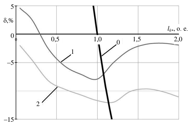
Рис. 6. Относительные погрешности определения I_{k*} при R_{пер} = 2R_{пер,задан} , S_{сист} = 2S_{задан} ; I_{нагр} = I_{нагр,мах} , I'_{k(0)} = 1,1I_{k(0)} , I'_{k(2)} = 1,1I_{k(2)} ; 0 – кривая предельных погрешностей; 1 – при трехфазном КЗ; 2 – при двухфазном КЗ
