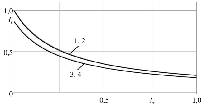
Рис. 2. Кривые спахания токов КЗ: 1, 2 – реальные и расчетные токи при трехфазных КЗ; 3, 4 – то же при двухфазных КЗ
