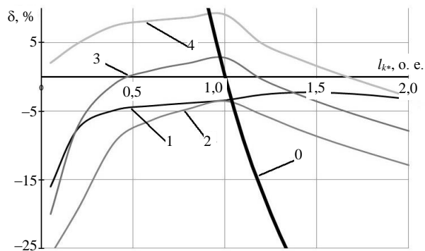
Рис. 5. Относительные погрешности определения l_{k^*} при трехфазном КЗ с учетом погрешностей расчета токов КЗ ( I'_{k(0)} , I'_{k(1)} , I'_{k(2)} ) в начале и в конце защищаемых участков: 0 – кривая предельных погрешностей; 1 – при I'_{k(0)} = I_{k(0)} , I'_{k(1)} = I_{k(1)} , I'_{k(2)} = I_{k(2)} ; 2 – при I'_{k(0)} = 0,9I_{k(0)} , I'_{k(1)} = I_{k(1)} , I'_{k(2)} = 0,9I_{k(2)} ; 3 – при I'_{k(0)} = 0,95I_{k(0)} , I'_{k(1)} = 1,05I_{k(1)} , I'_{k(2)} = 0,95I_{k(2)} ; 4 – при I'_{k(0)} = I_{k(0)} , I'_{k(1)} = 1,1I_{k(1)} , I'_{k(2)} = I_{k(2)}
