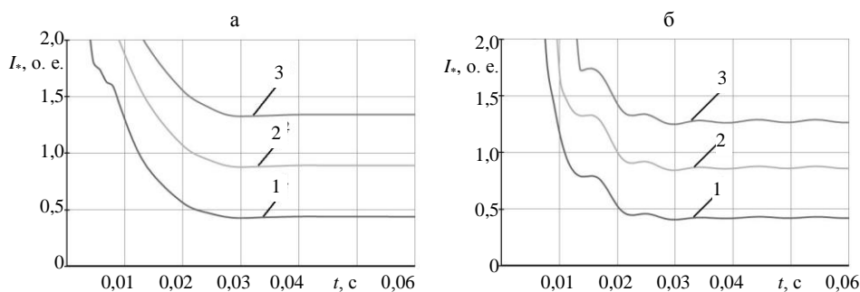
Рис. 8. Динамические характеристики работы ОМП при трех- (а) и двухфазном (б) КЗ и I_{\text{нагр}} = I_{\text{нагр.макс}} : 1 – при l_* = 0,5 ; 2 – 1,0; 3 – 1,5
