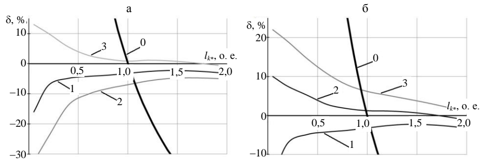
Рис. 4. Относительные погрешности определения l_{k^*} при трехфазном КЗ: 0 – кривая предельных погрешностей; а – при различных мощностях системы: 1 – при S_{сист} = S_{задан} ; 2 – при S_{сист} = 2S_{задан} ; 3 – при S_{сист} = 0,5S_{задан} ; б – при различных величинах переходного сопротивления: 1 – при R_{пер} = 0 ; 2 – при R_{пер} = R_{пер.задан} ; 3 – при R_{пер} = 2R_{пер.задан}
