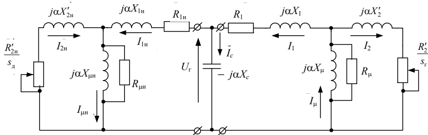
Рис. 2. Схема замещения системы АГ–ЕСВ–АД
