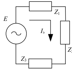
Рис. 4. Эквивалентная схема замещения системы АГ-ЕСБ-АД
