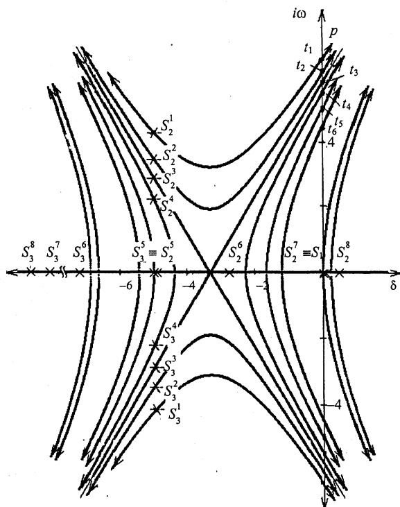
Рис. 2. Фрагмент корневого портрета интервальной динамической системы, описываемой характеристическим полиномом p^3 + a_1 p^2 + a_2 p + a_3 при 40 \leq a_2 \leq -5
