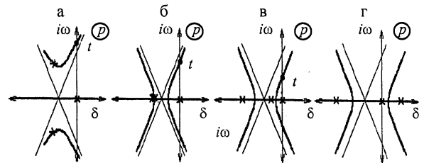
Рис. 1. Динамика корневого портрета при непрерывном изменении коэффициентов характеристического уравнения на заданных интервалах
